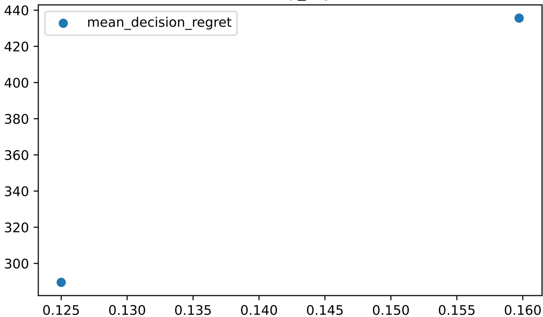
accuracy_regret
