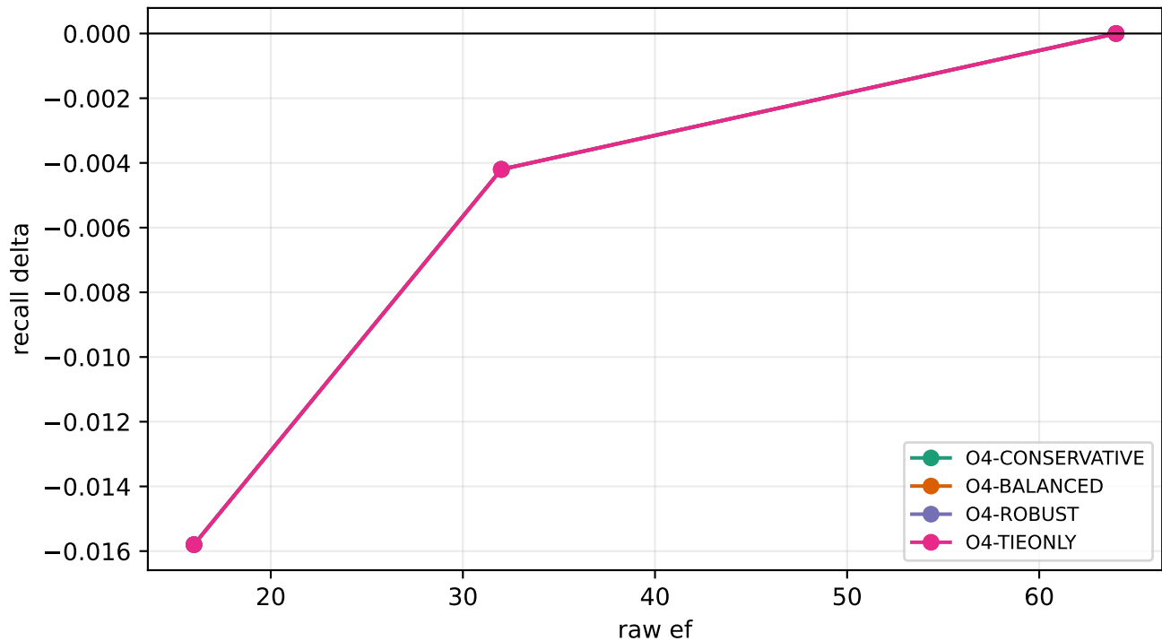
O4 recall delta vs O0
