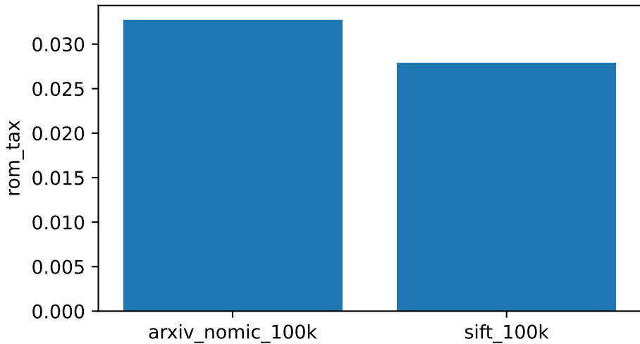
Robustness
