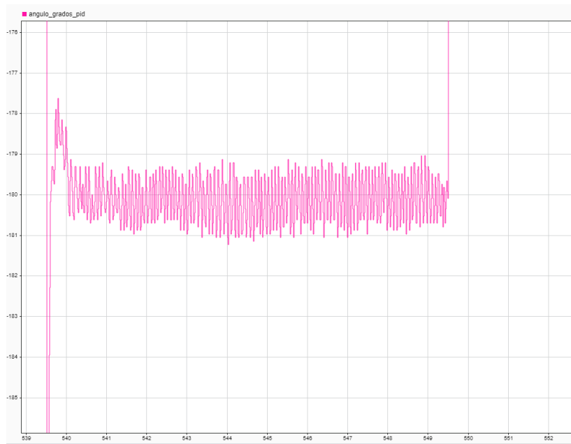
Figura 18: 3 reducido angulo
