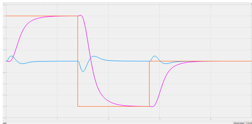
Figura 9: 3 reducido sim
