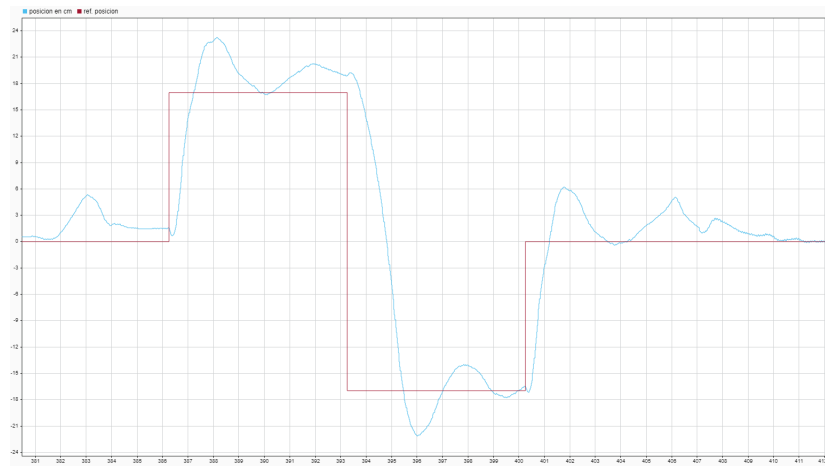
Figura 1: 1 PID pos
