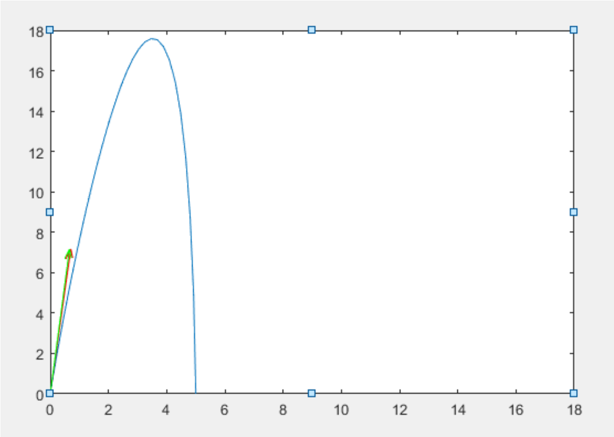
Figura 5: Trayectoria X_2 vs X_1 respuesta natural con condiciones iniciales (4, 0)
