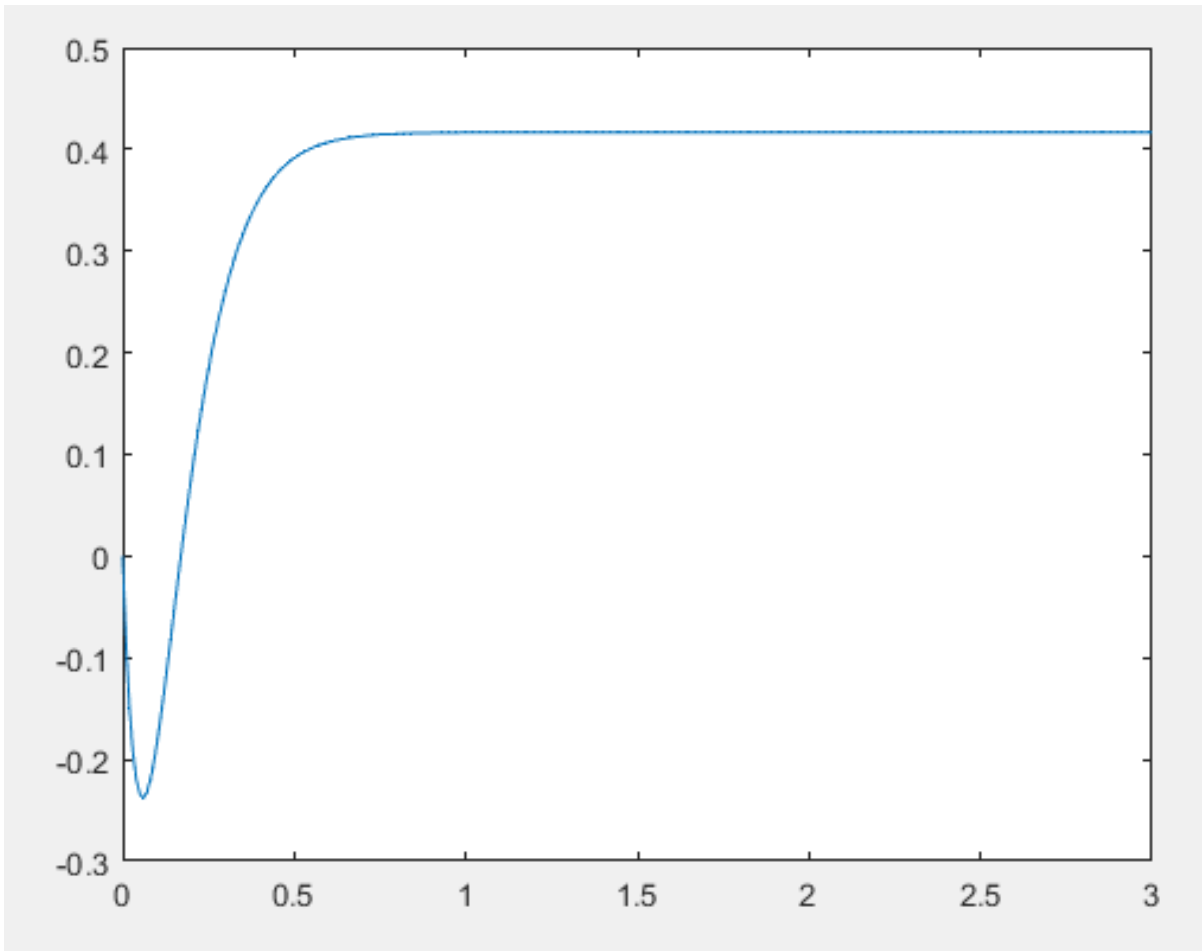
Figura 13: Respuesta del sistema usando la salida reconstruida W \cdot D
