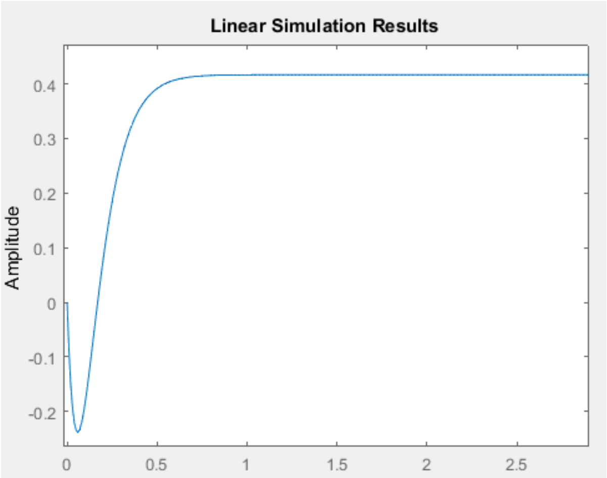
Figura 2: Respuesta a la entrada escalón
