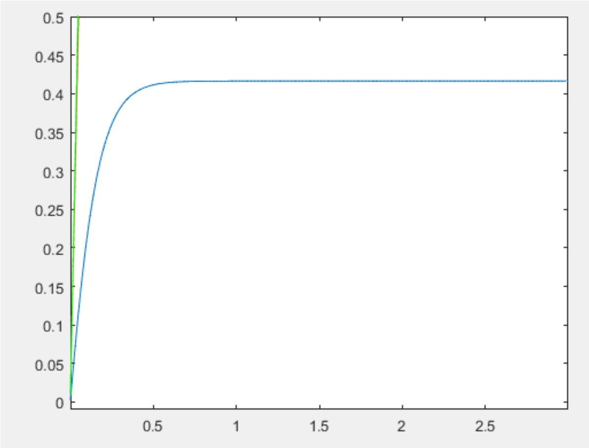
Figura 15: Comportamiento del estado X_1 vs tiempo del sistema originalmente
