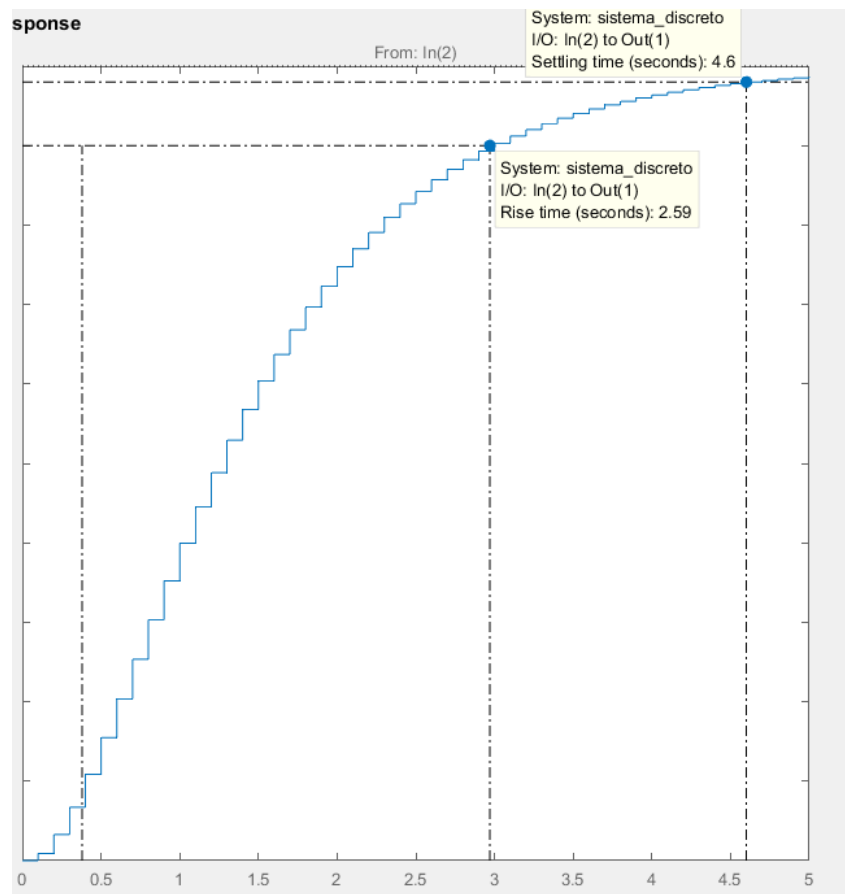
Figure 1: Respuesta en tiempo del sistema en lazo abierto.
