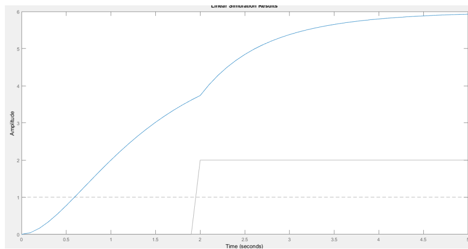
Figure 2: Respuesta en tiempo del sistema en lazo abierto con perturbación en t=2 .
