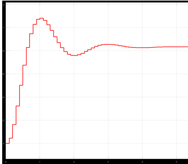
Figure 3: Respuesta en tiempo del sistema en lazo cerrado ( K_p=1 , K_i=0 , K_d=0 , T_d=0 ).
