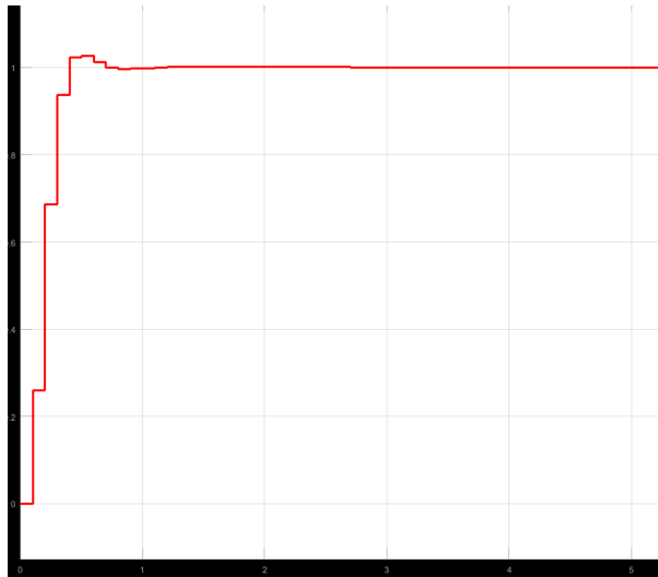
Figure 4: Respuesta en tiempo del sistema en lazo cerrado ( K_p=1.45 , K_i=1 , K_d=0.43 , T_d=0 ).
