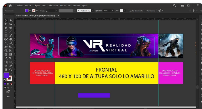
Especificación para gran formato — despiece del banner en frontal y laterales, con medidas en centímetros anotadas para el instalador.
