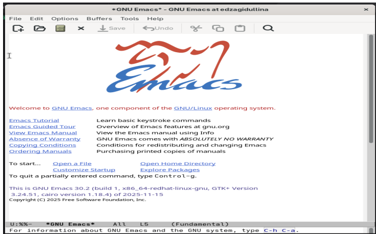
Рисунок 1: Запуск Emacs
