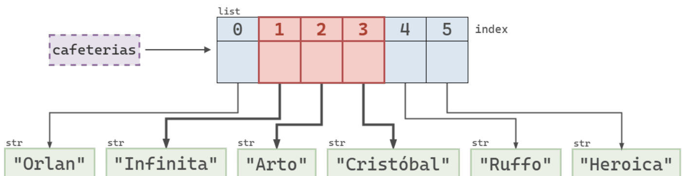
Figura 3: Selección de sublista de cafeterías usando el slice 1:4 .
