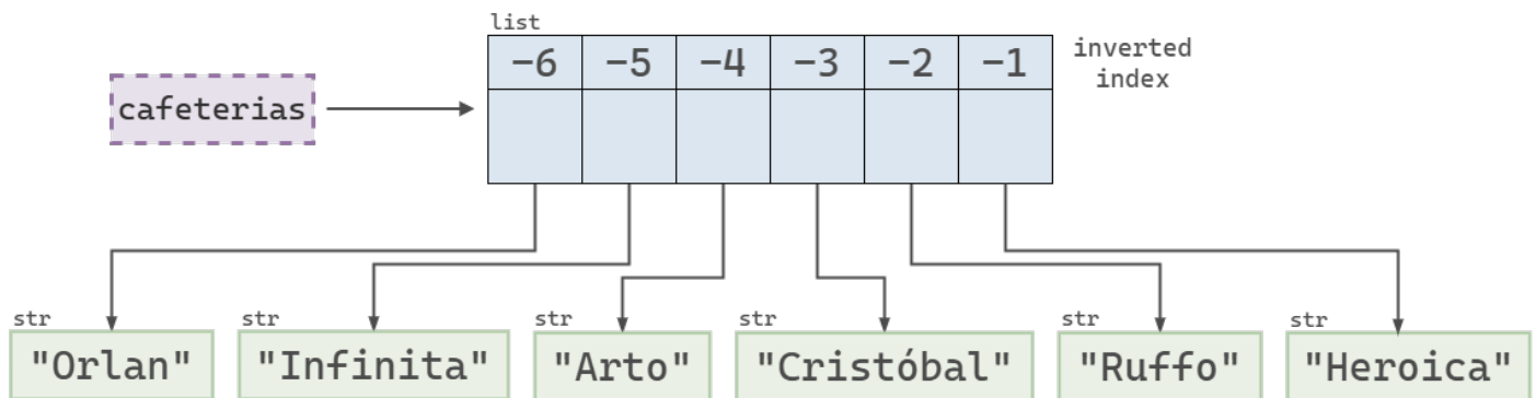
Figura 2: Representación gráfica de cafeterias utilizando índices negativos para cada elemento.
