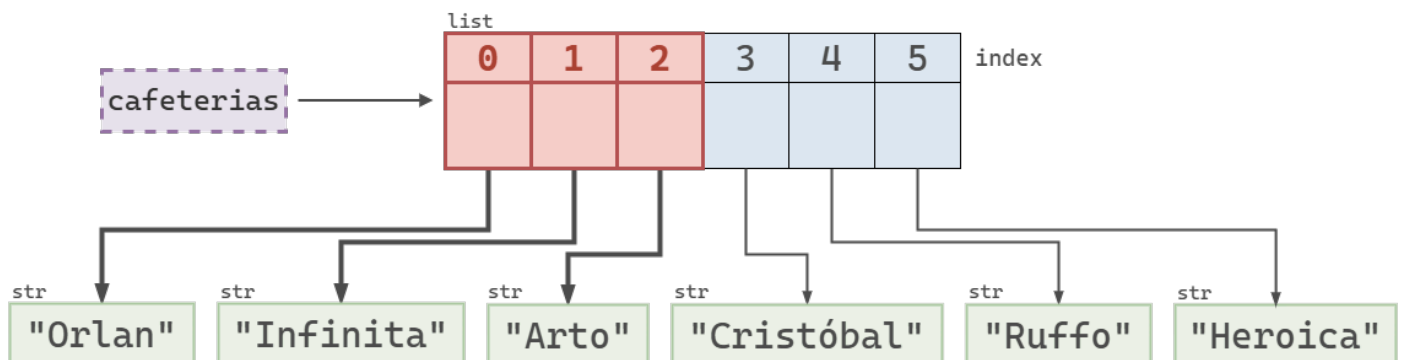
Figura 5: Selección de sublista de cafeterias hasta el índice 3 usando el slice de inicio implícito :3 .
