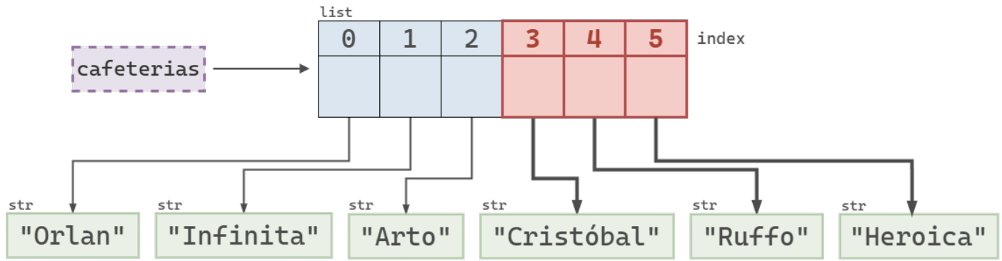
Figura 6: Selección de sublista de cafeterias desde el índice 3 usando el slice con fin implícito 3:.
