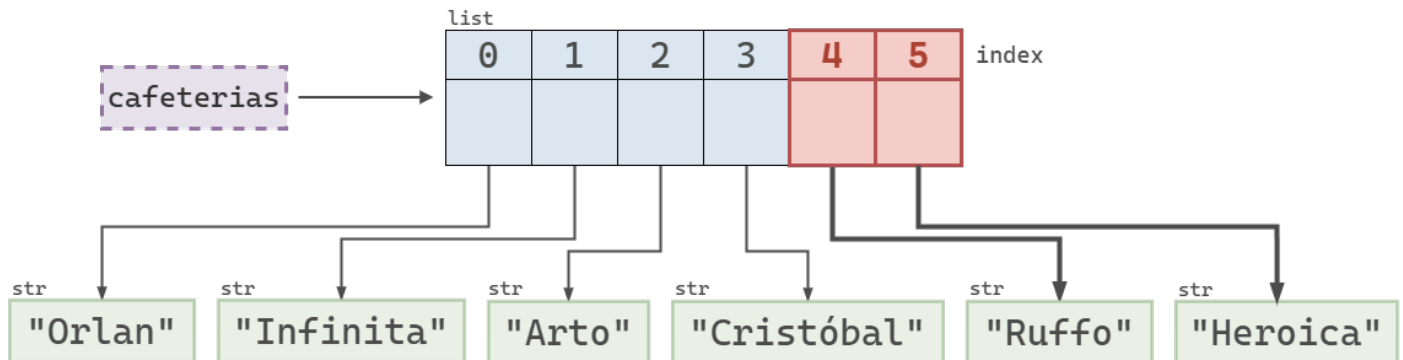
Figura 4: Selección de sublista de cafeterias usando el slice 4:6.
