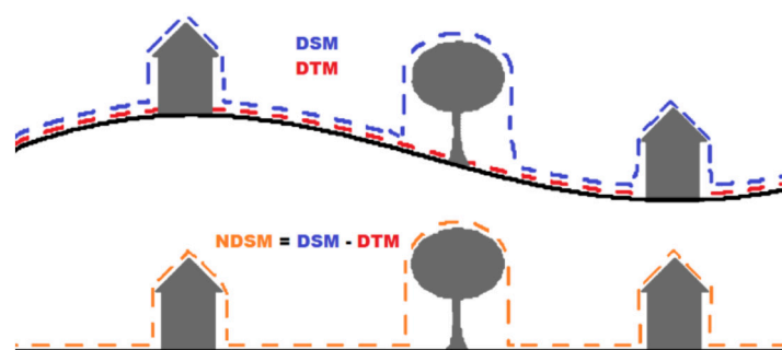
Figure 4: DSM computation principle ( http://www.stadtentwicklung.berlin.de/umwelt/umweltatlas/ed610_03.htm )
