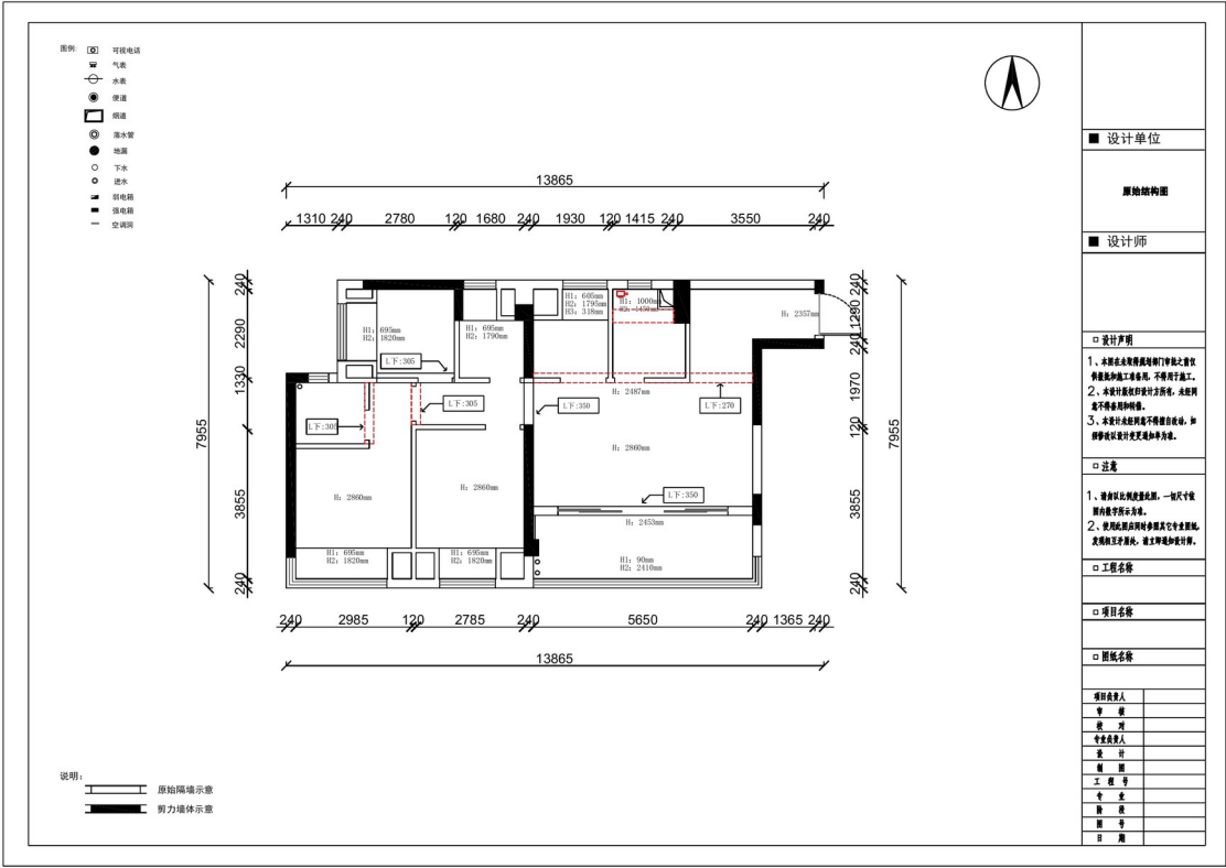
图：D10 原始户型图旋转便读版。图中红色虚线为拆改/调整标注，实际施工需由设计师、物业和施工方复核。
