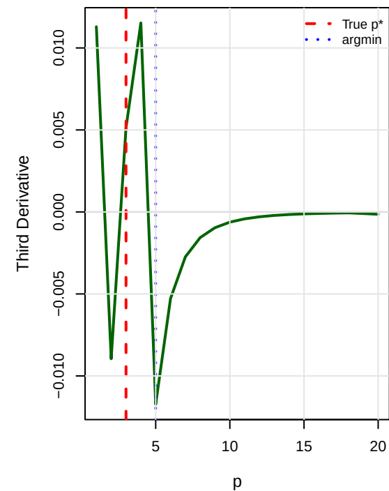
\Delta_3
