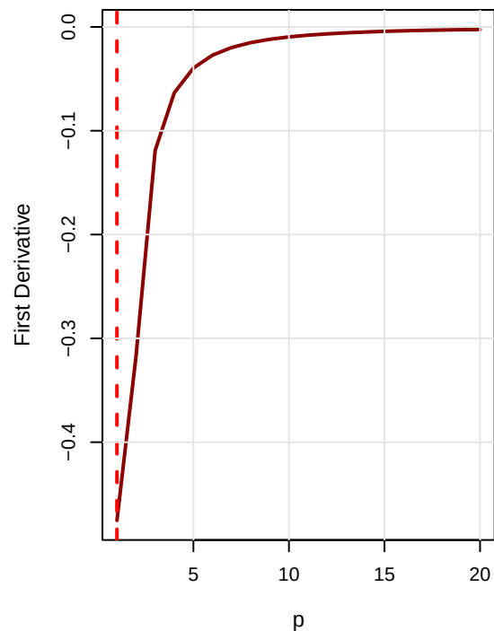
\Delta_1
