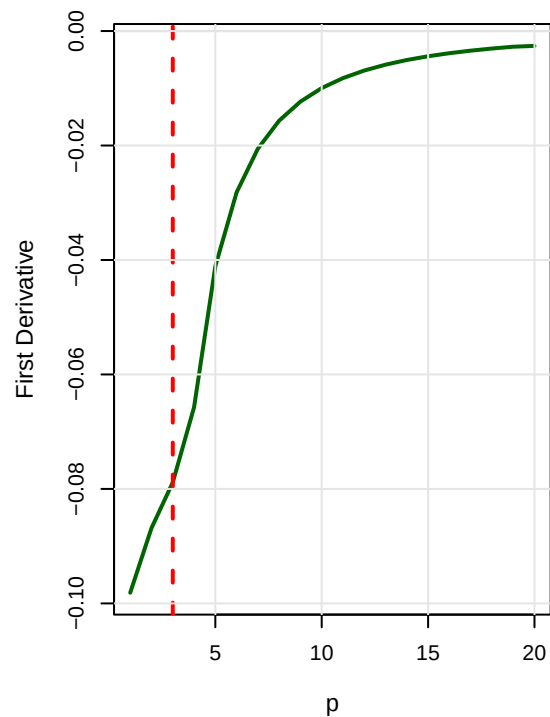
\Delta_1
