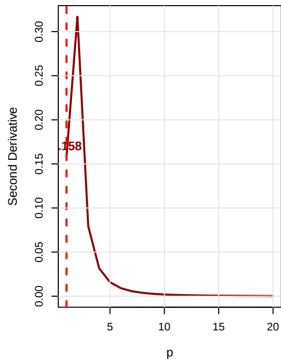
\Delta_2
