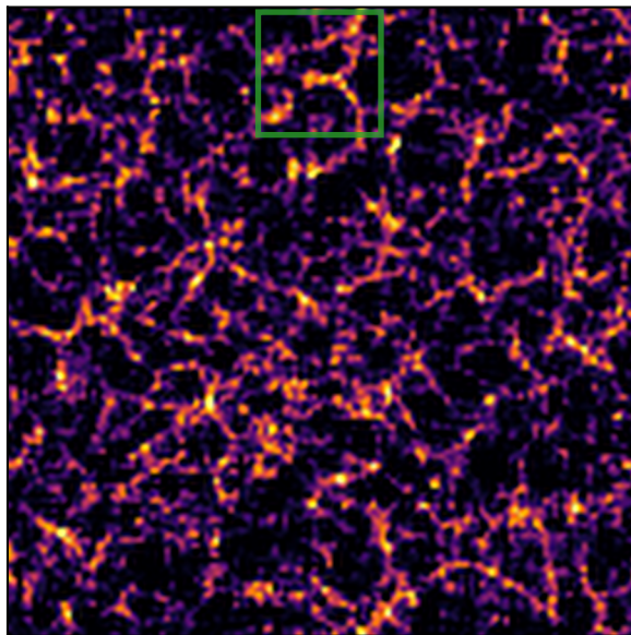
GADGET-4
