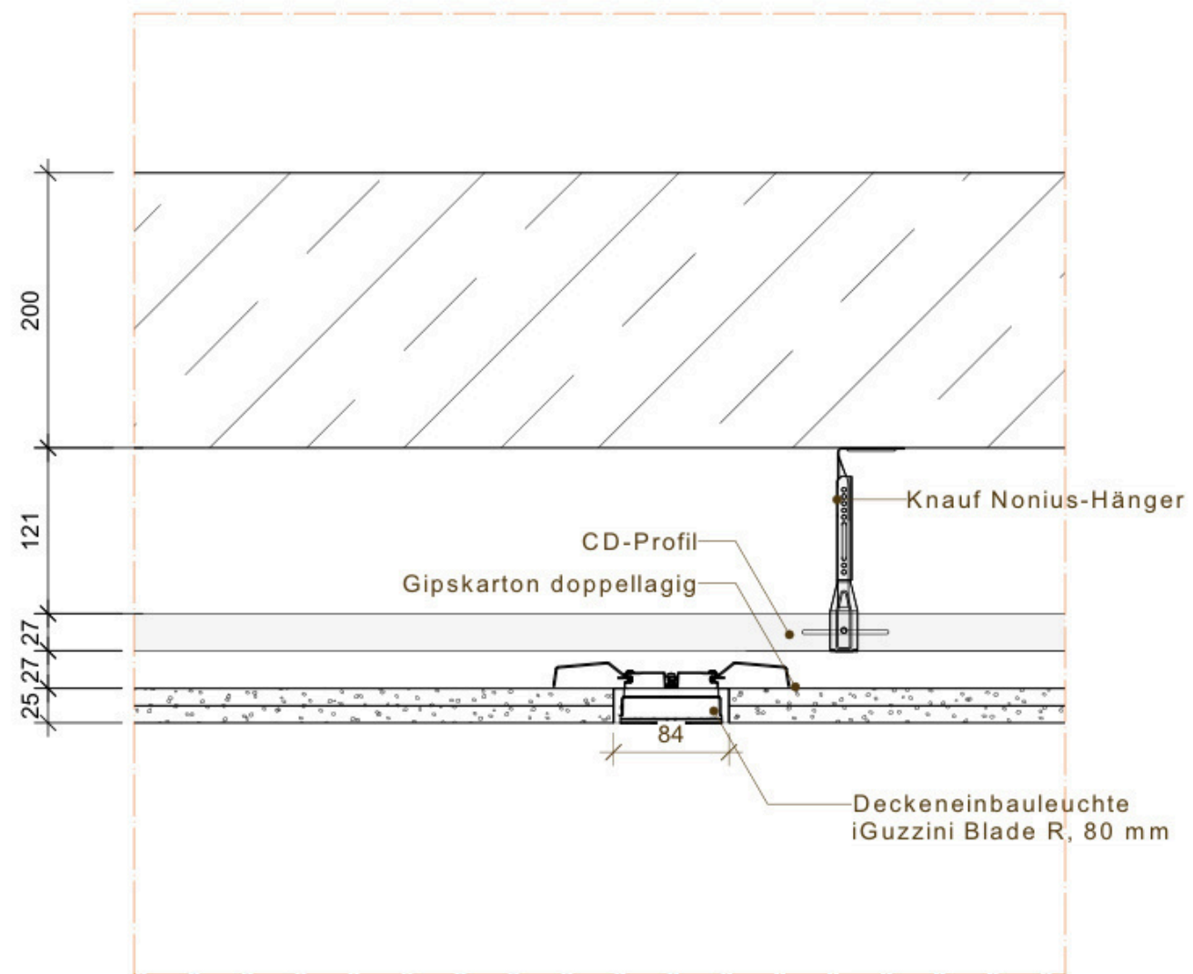
Deckeneinbauleuchte Detail M 1:5
