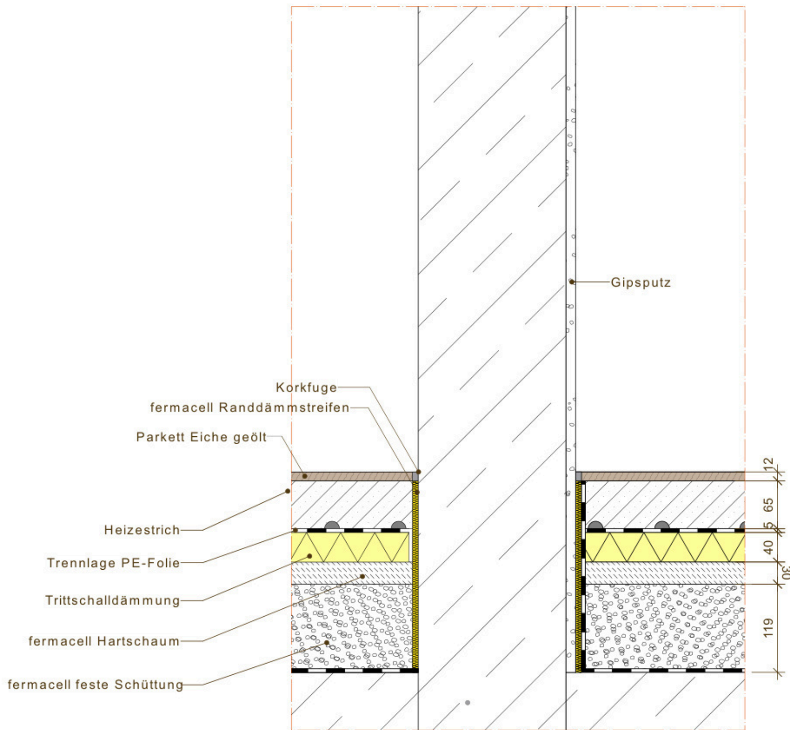
Tragende Wand- Boden Detail 4 M 1:5
