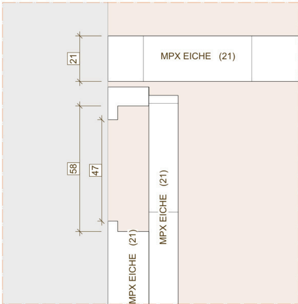
Griffmulde Detail 5 M 1:5
