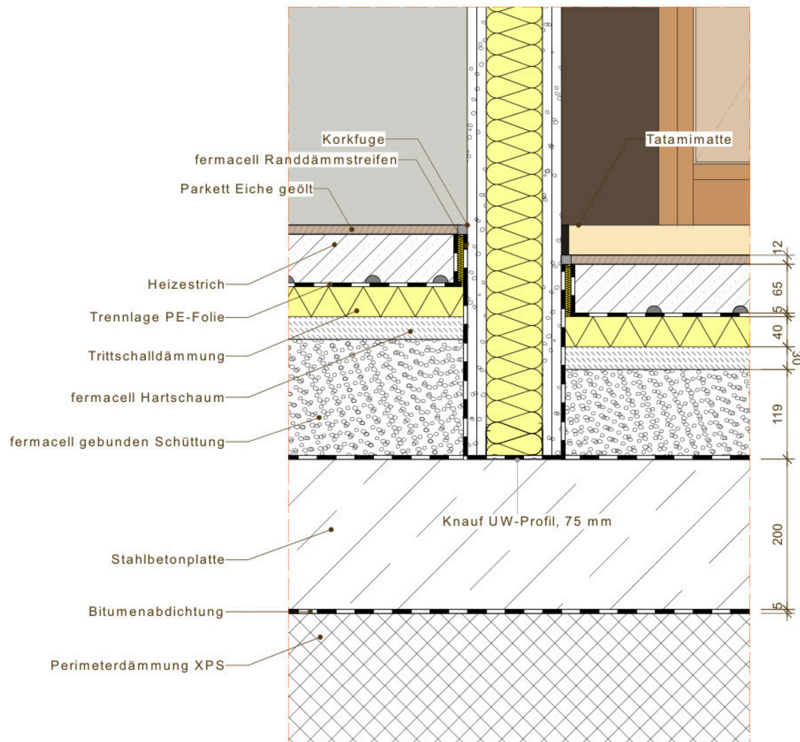
Bodenwandanschluss Detail 1 M 1:5
