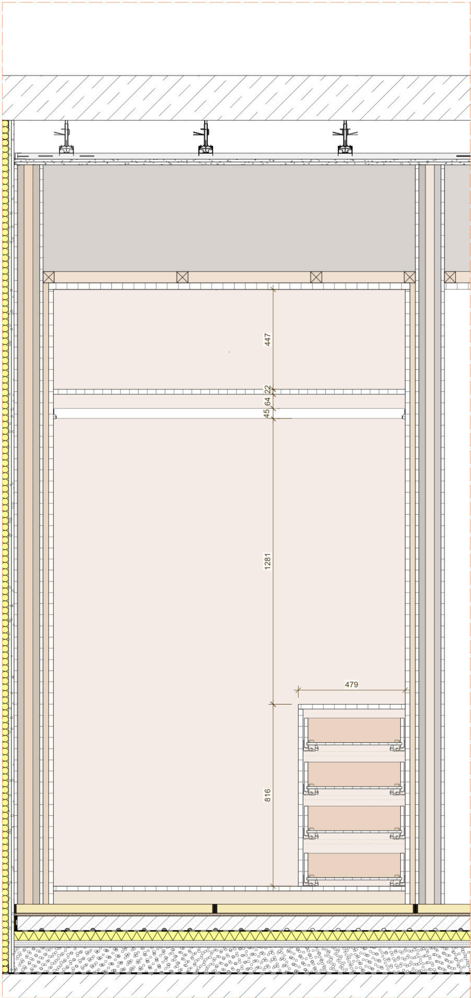
Einbauschränke Schnitt F-F' M 1:10
