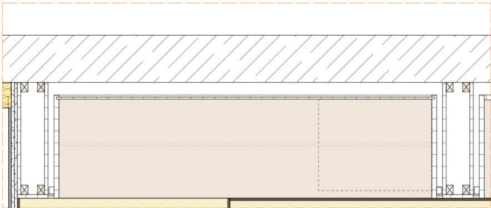
Einbauschränke Schnitt F-F' M 1:10
