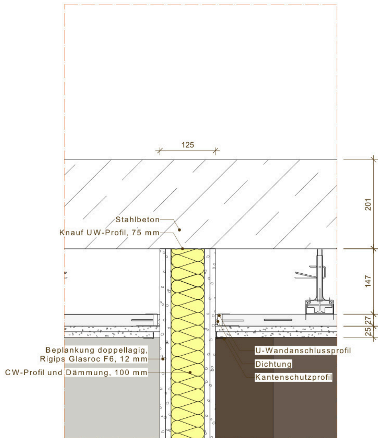
Deckenwandanschluss Detail 1 M 1:5
