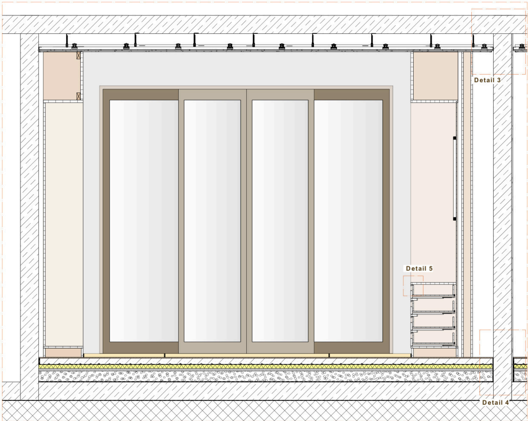
Querschnitt C-C' M 1:20
