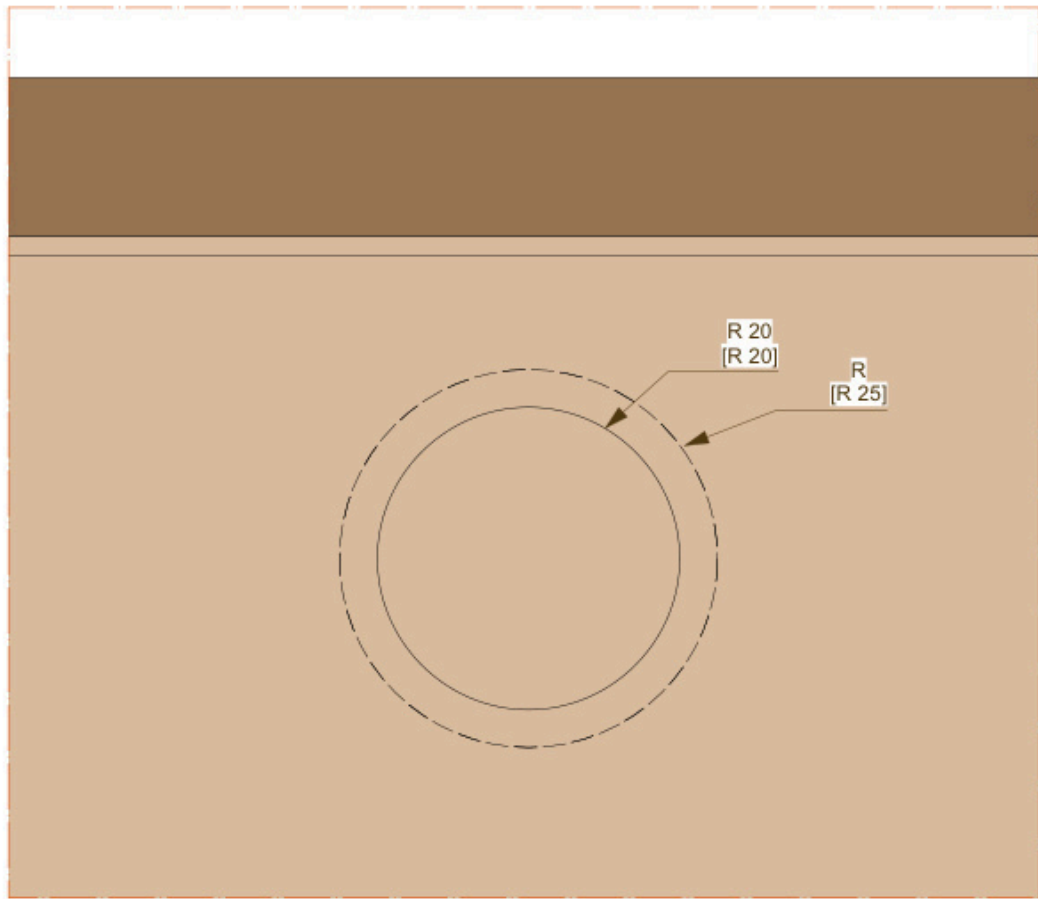
Griffmulde Detail 5 M 1:5
