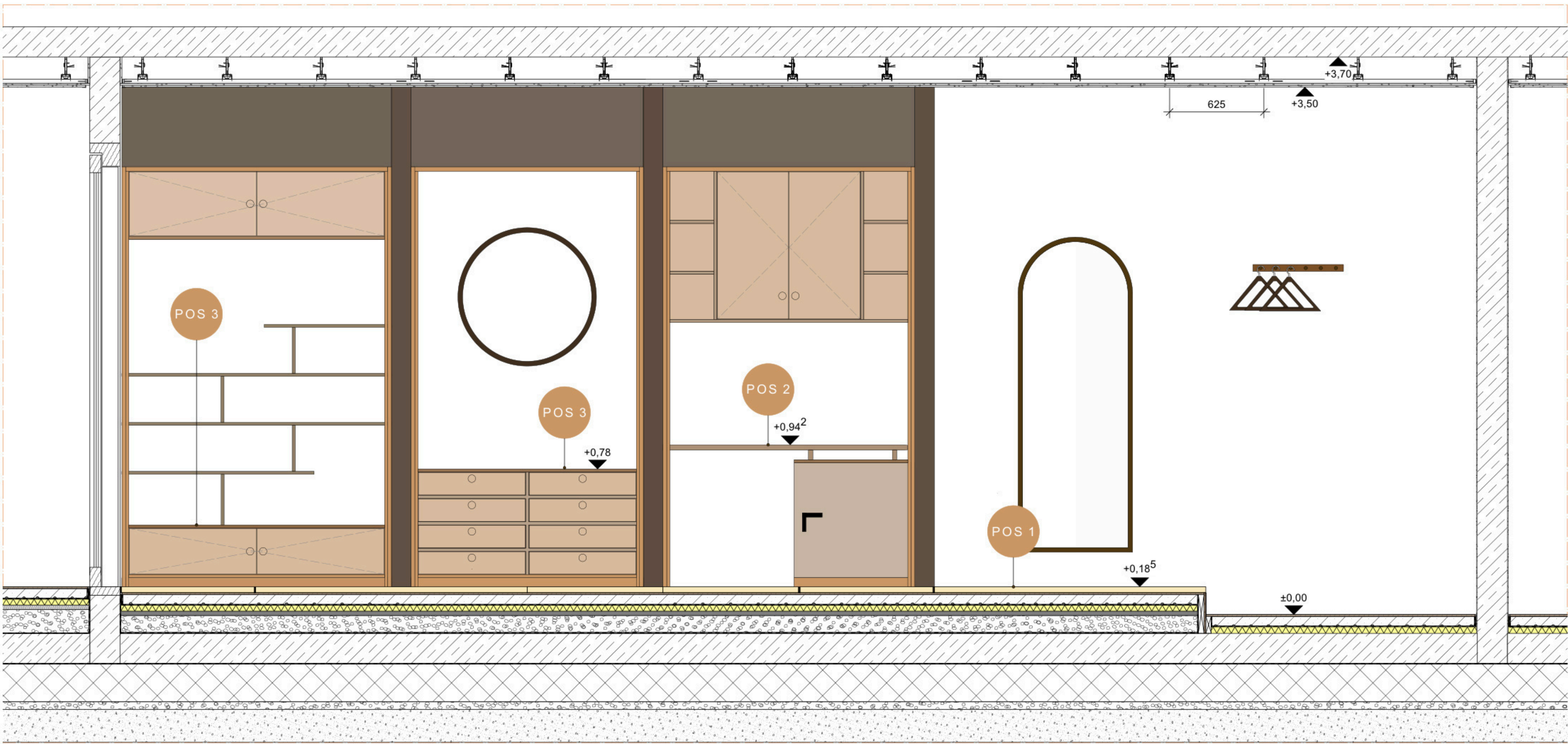
Längsschnitt A-A' M 1:20
