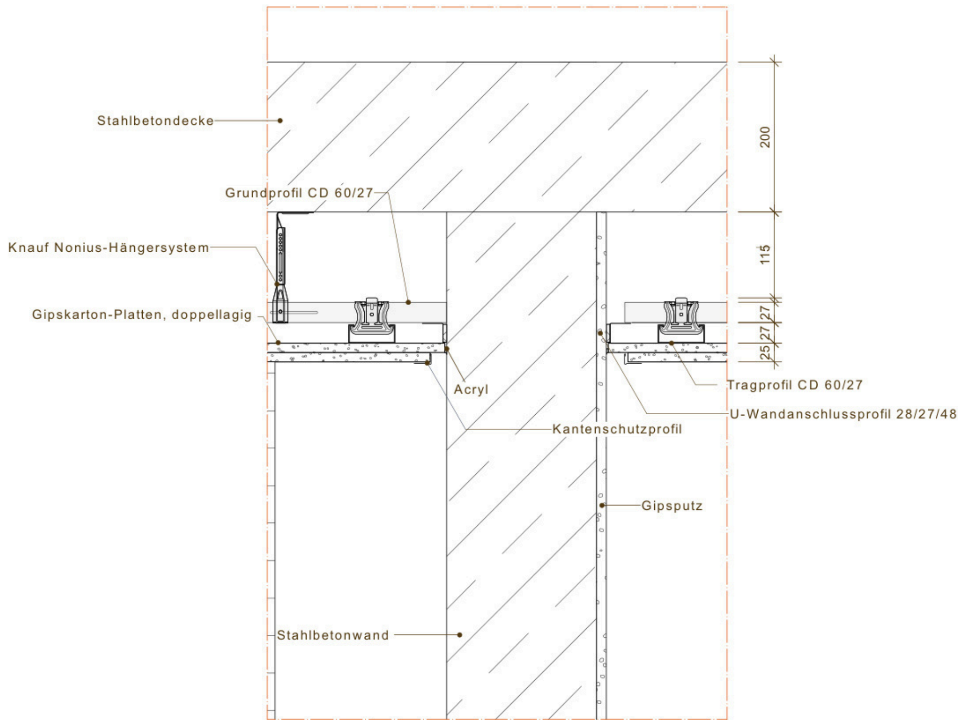
Abgehängte Decke Detail 3 M 1:5
