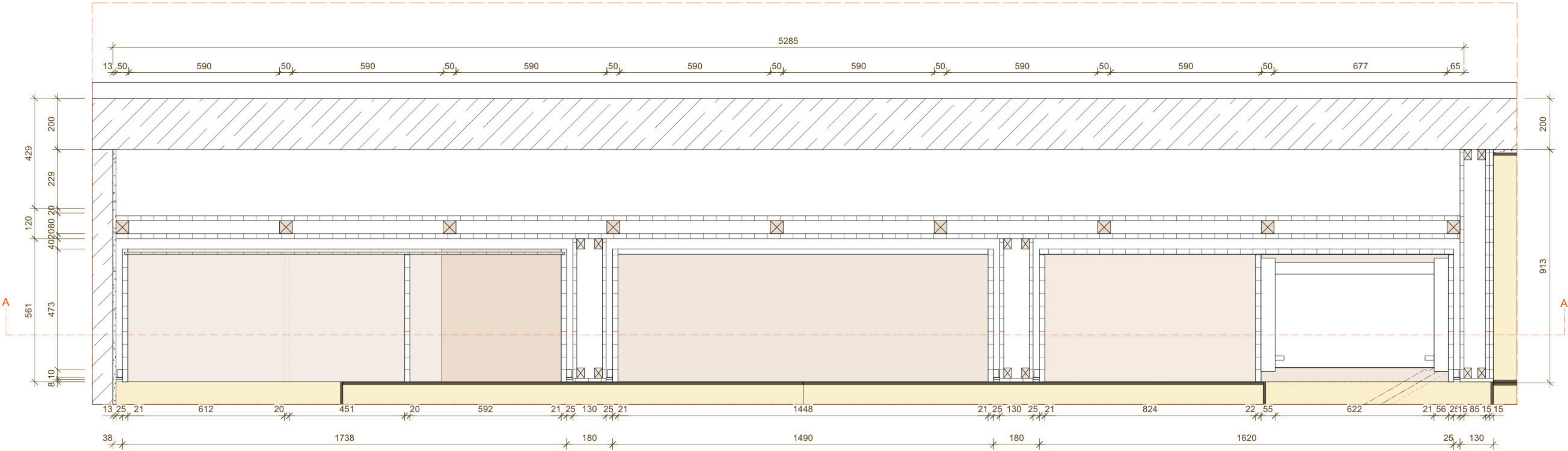
Einbauschränke Schnitt B-B' M 1:10
