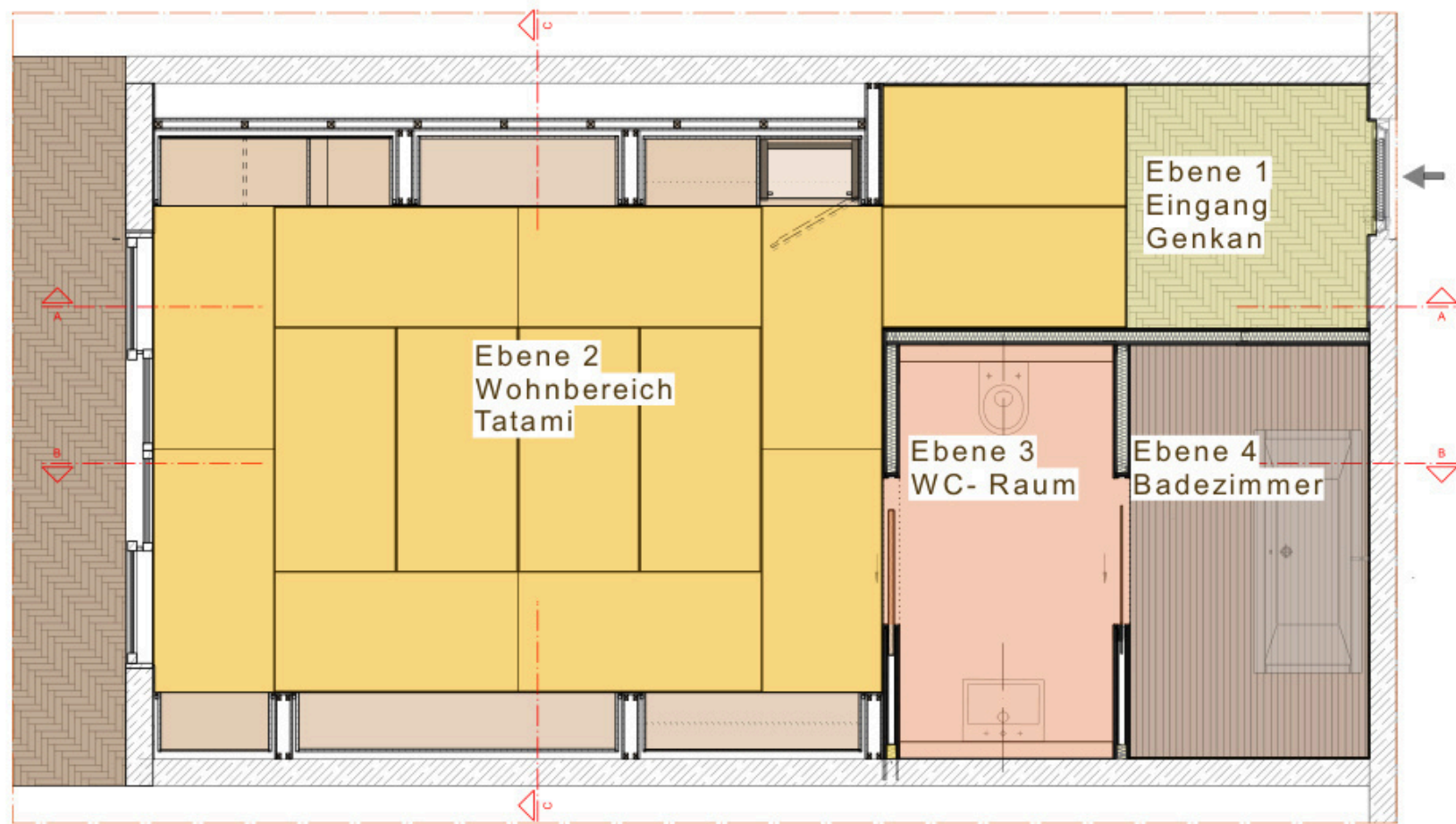
Bodenbelag Schema M 1:50
