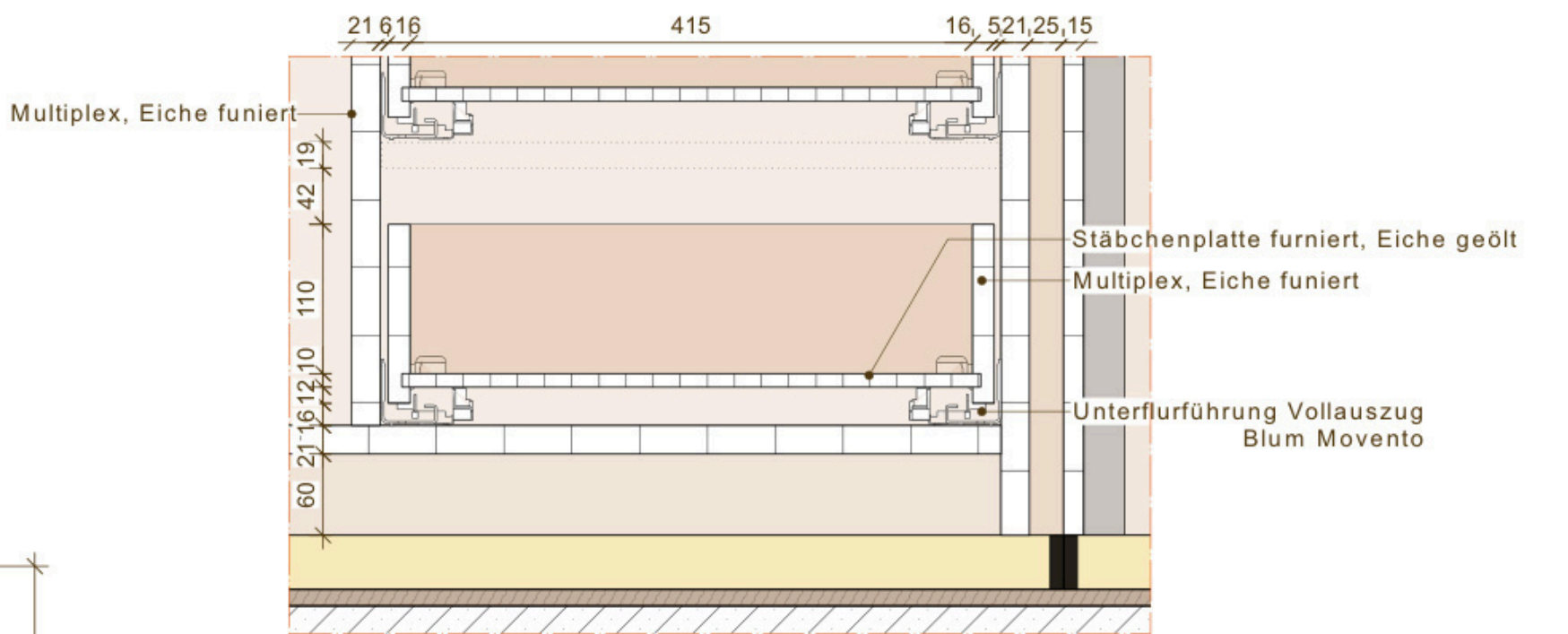
Schubladen Detail 6 M 1:5
