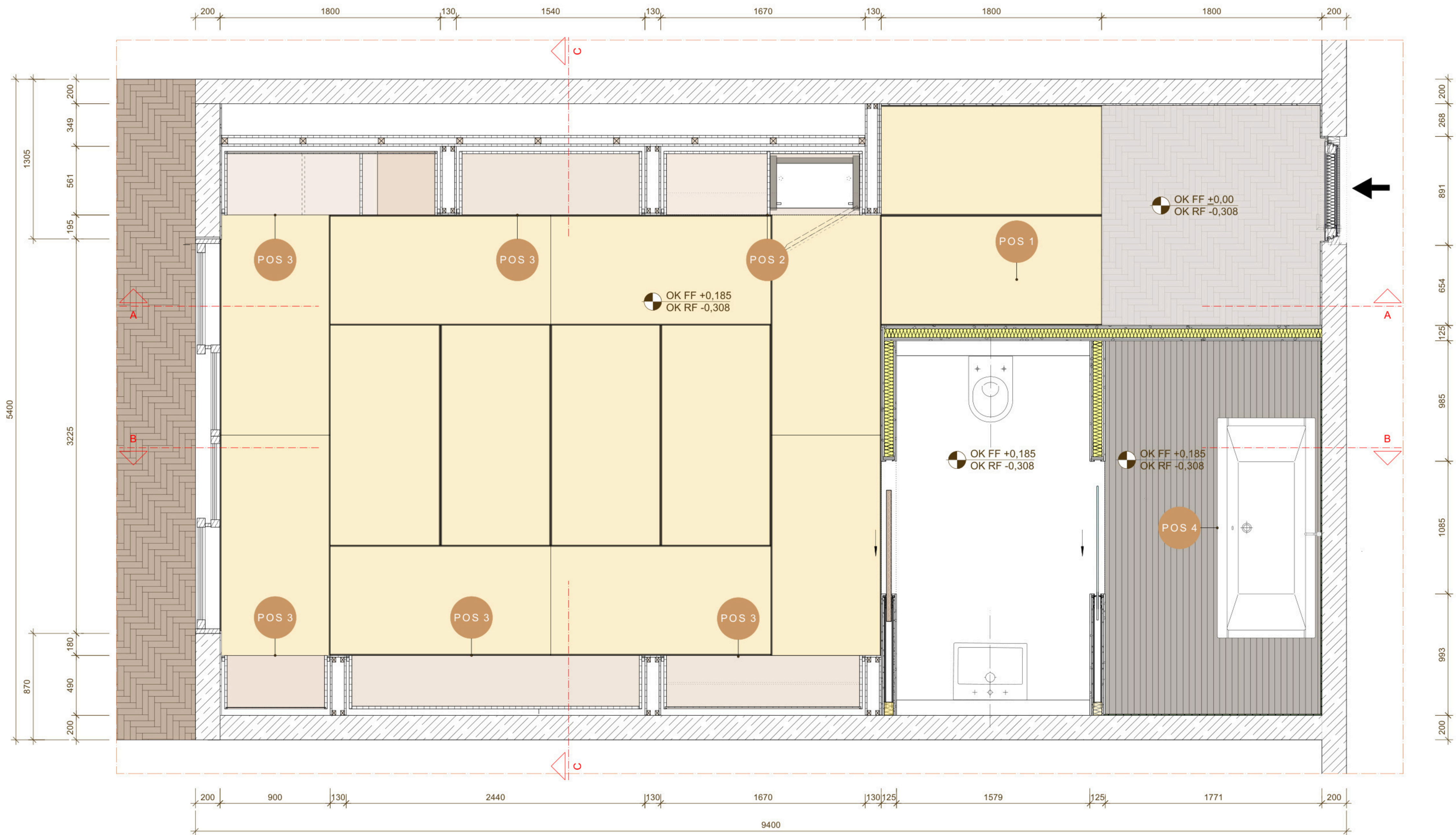
Grundriss M 1:20
