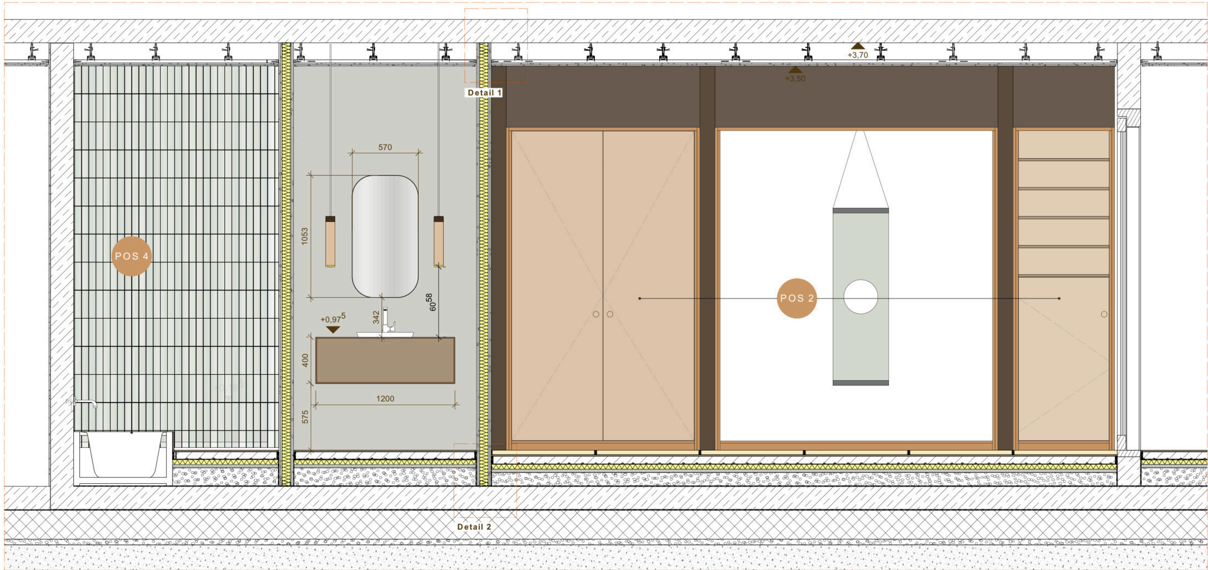
Längsschnitt B-B' M 1:20
