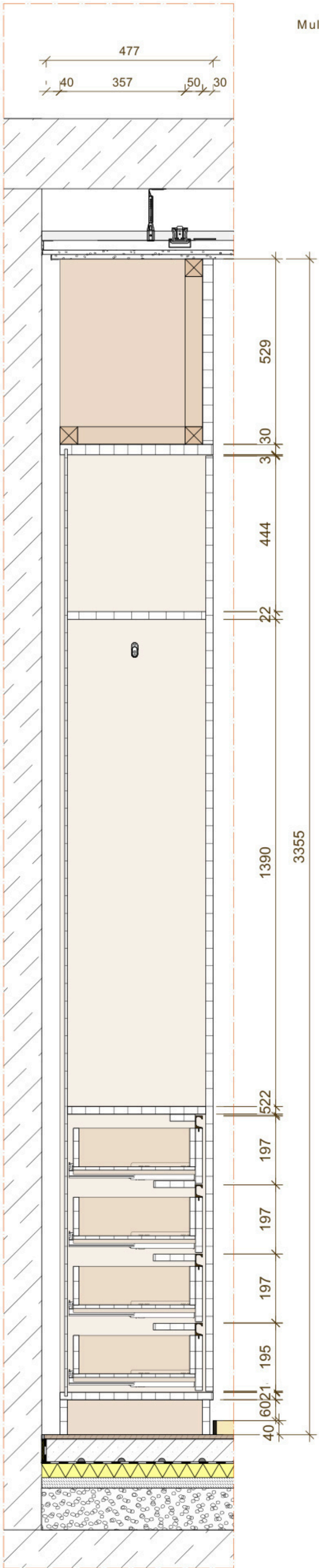
Einbauschränke Schnitt G-G' M 1:10
