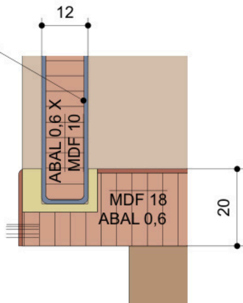
Detail Führungsschiene M1:1
