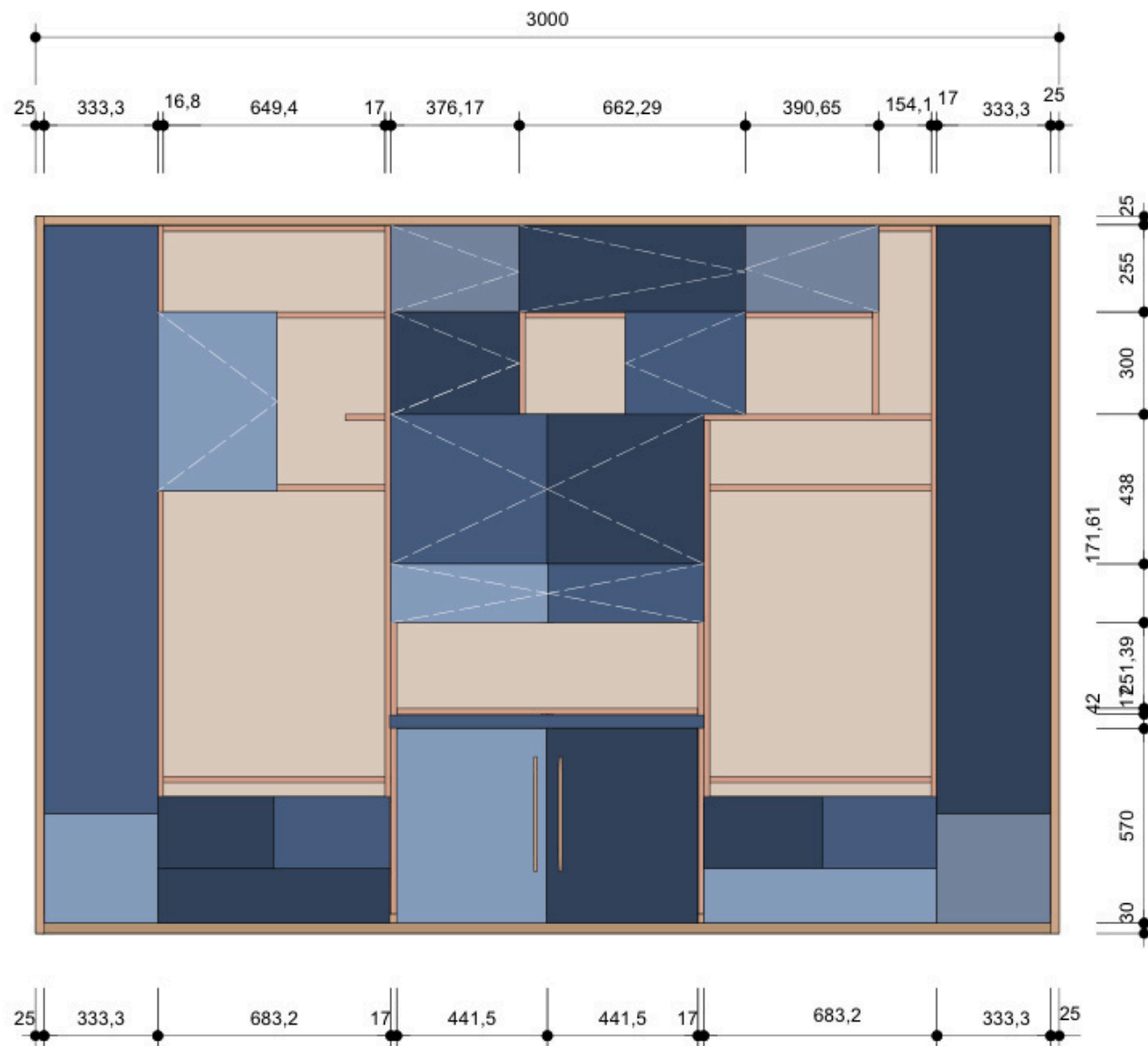
Ansicht M1:20
