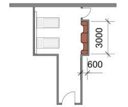
Grundriss M1:100
