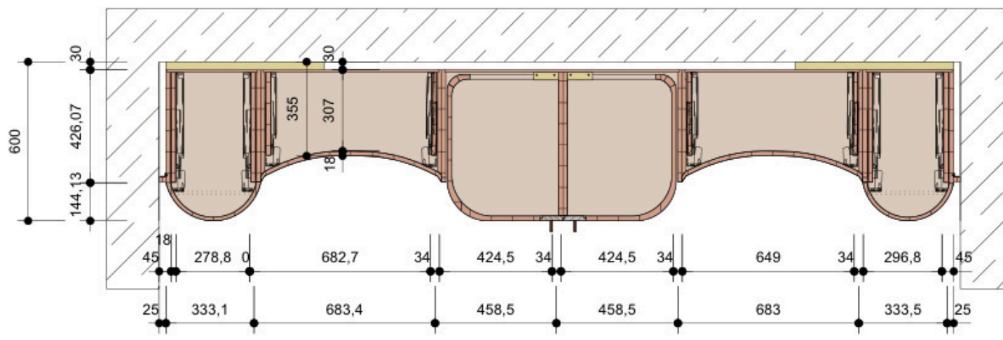
Schnitt CC M1:20
