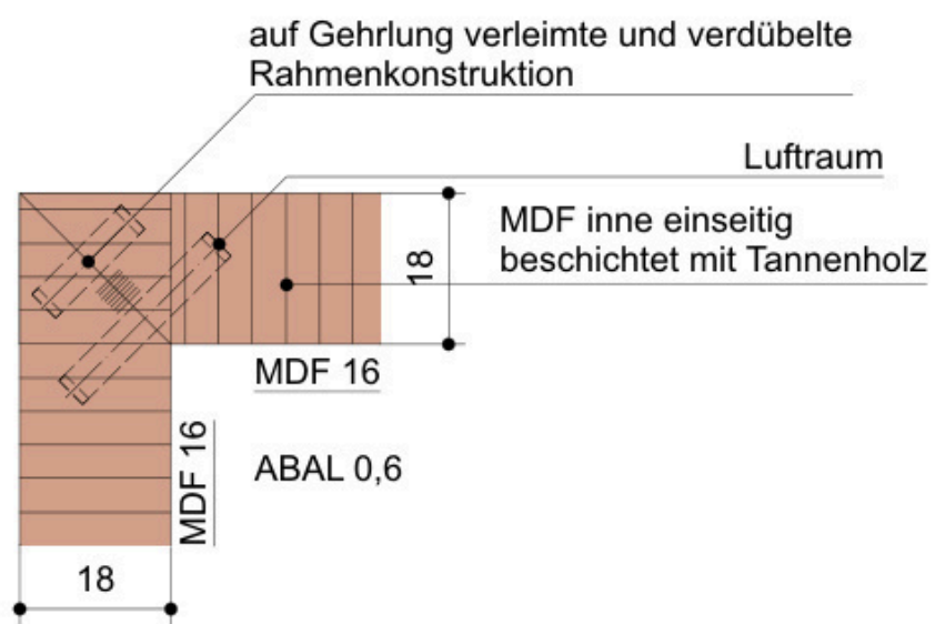
Detail Eckverbindung M1:1
