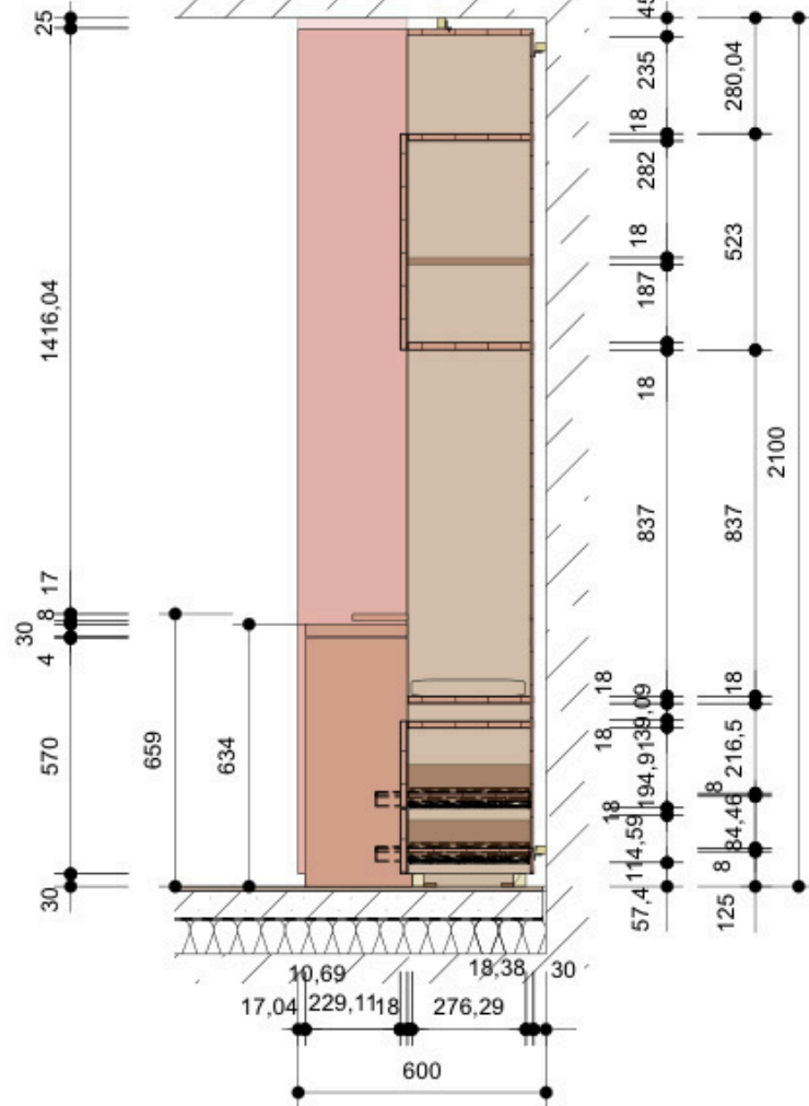
Schnitt AA M1:20
