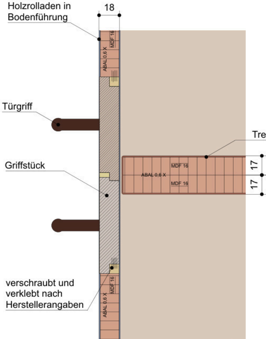
Detail Türgriff M1:2
