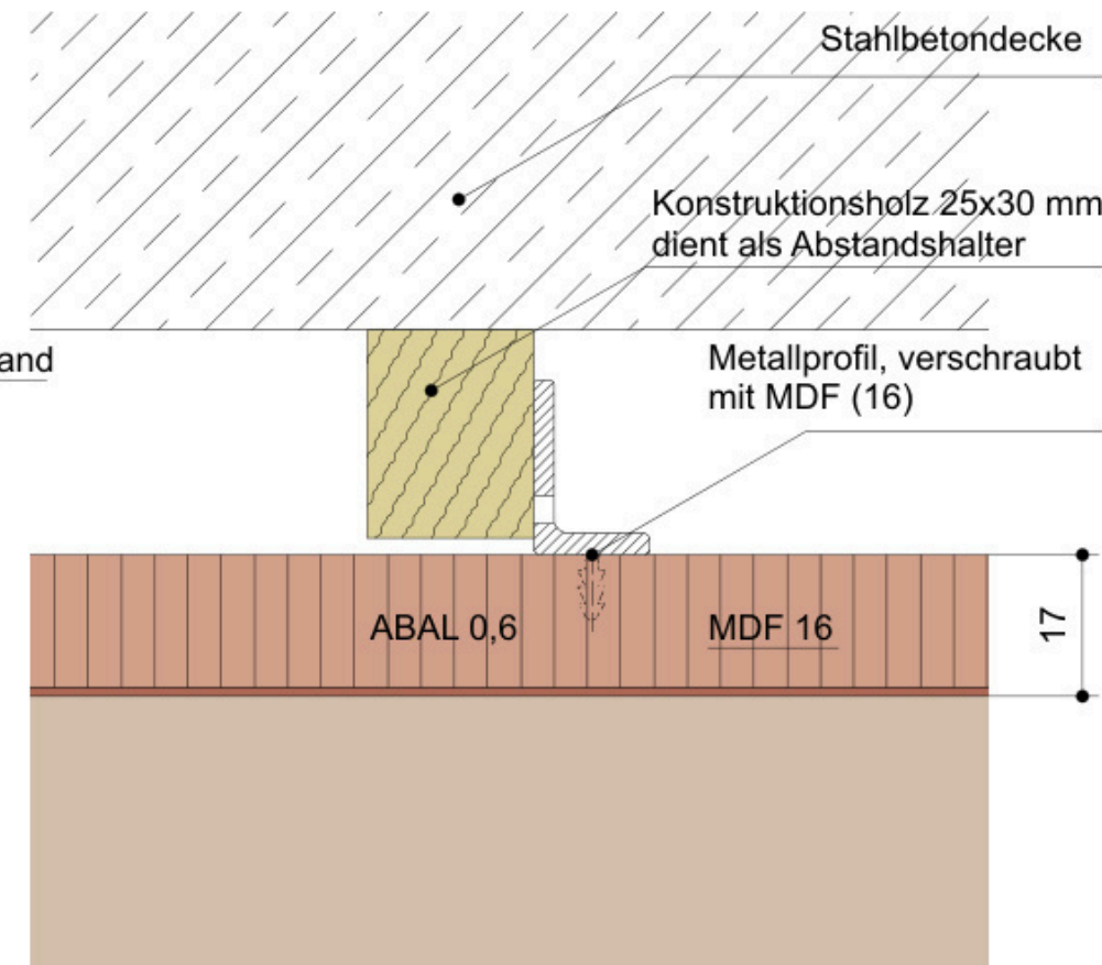
Detail Möbelrahmen M1:1
