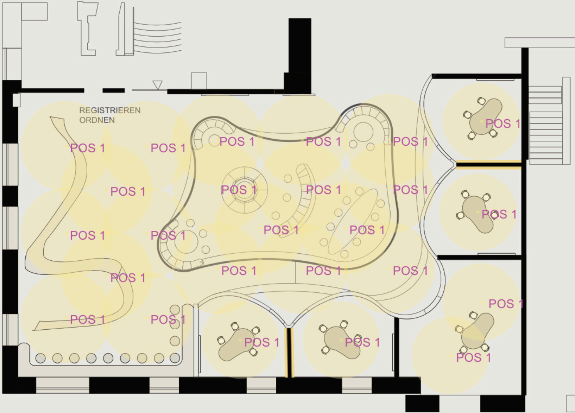
Grundbeleuchtung im Grundriss M 1:200
