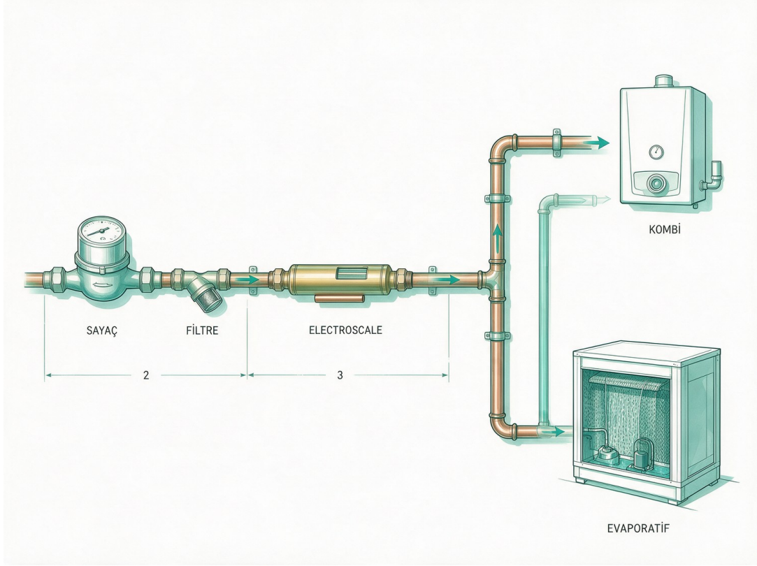
Tesisat bağlantı şeması: sayac → filtre → ElectroScale → kombi / evaporatif soğutucu
