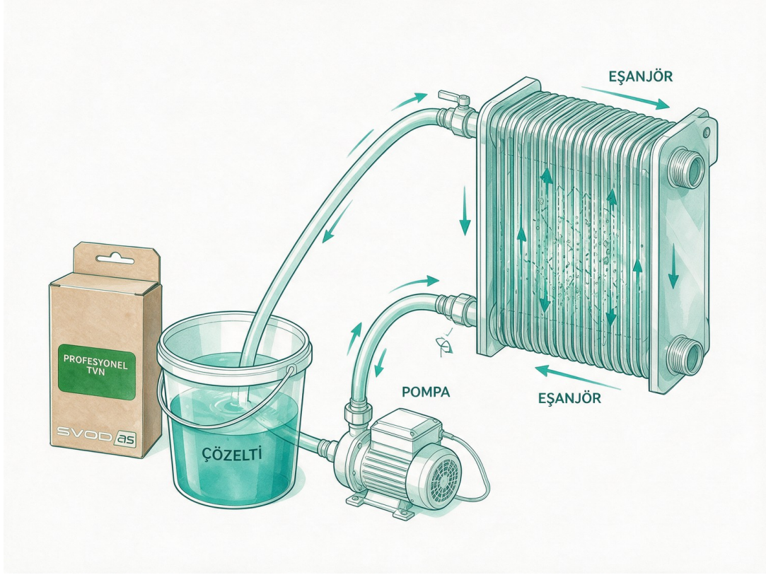
CIP sirkülasyon şeması: çözelti kabı → pompa → eşanjör → dönüş hattı (kapalı devre)
