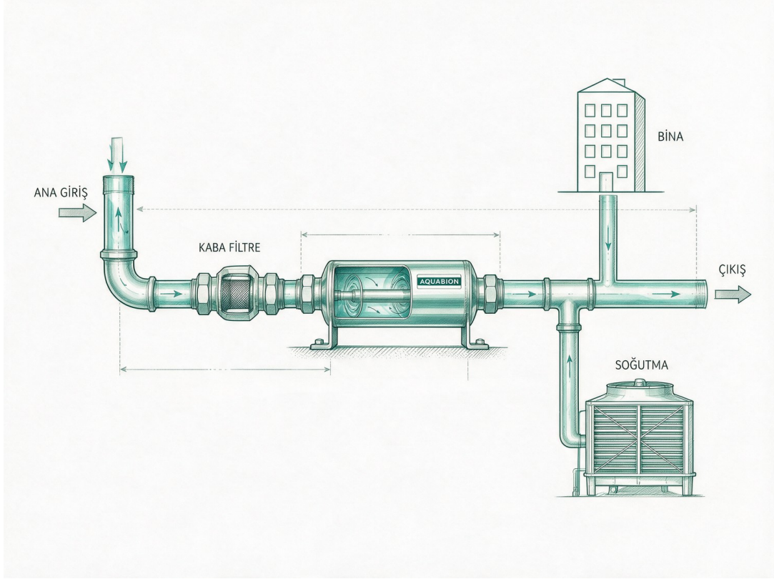
Tesisat bağlantı şeması: ana giriş → kaba filtre → Aquabion → bina / soğutma hatları
