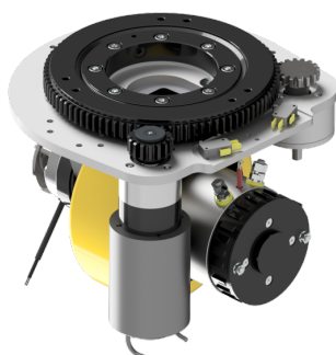
Figura 3.4: Render della motoruota MRT05 di CFR.
