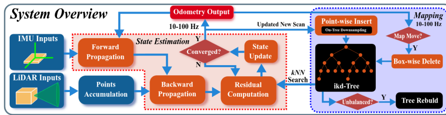
Figura 2.1: Diagramma a blocchi dell'algoritmo FAST-LIO 2. Adattato da [19].
