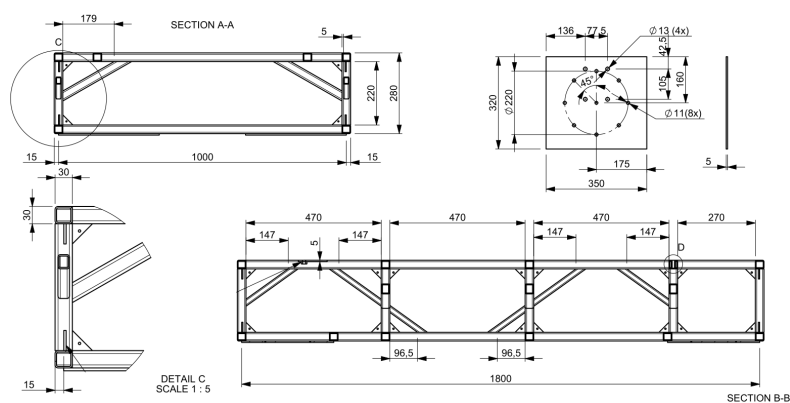
Figura 3.13: Progetto CAD del telaio del veicolo – quote significative.
