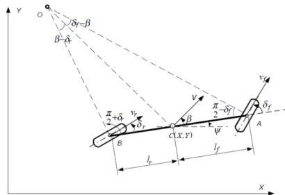
Figura 2: Modello a Biciclo Sterzante
