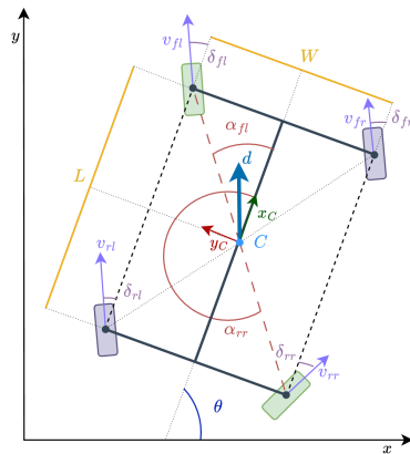
Figura 3: Ruote motrici in verde, passive in viola.
