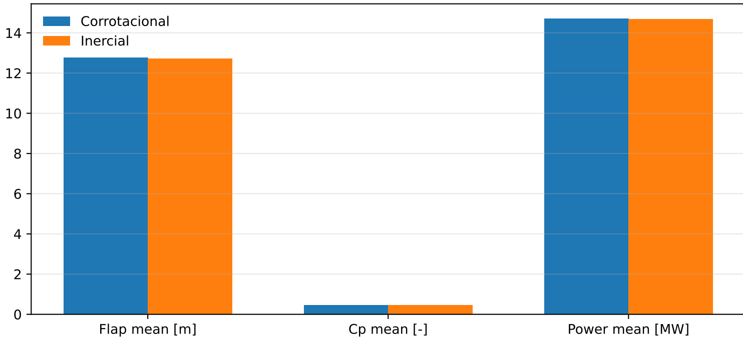
Comparación corrotacional vs inercial (yaw=0°)
