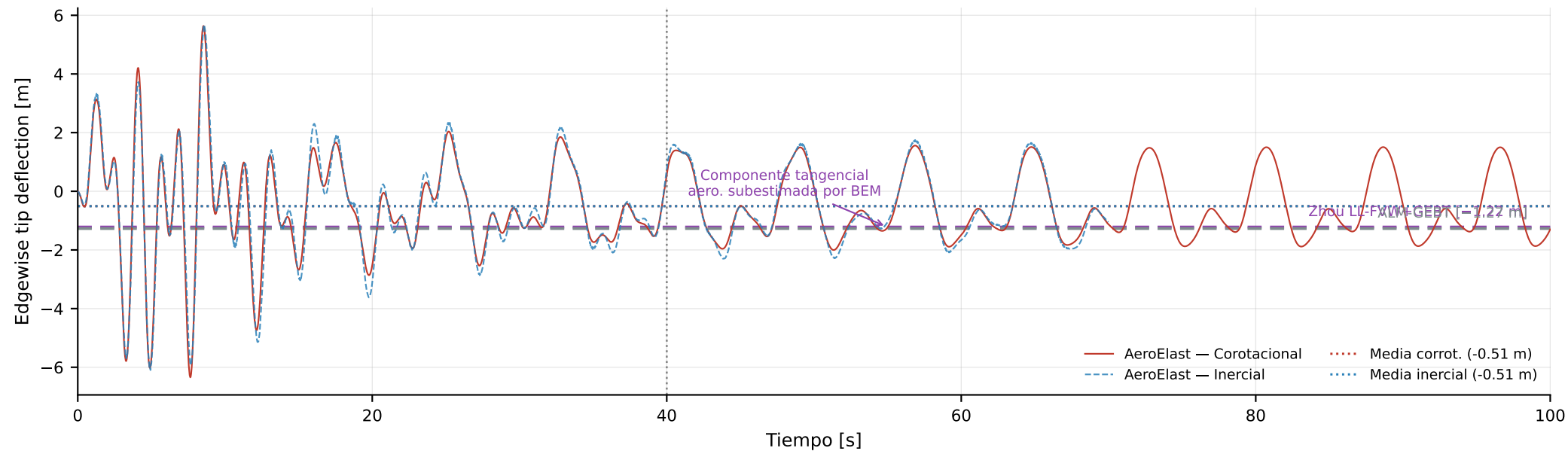
(b) Deflexión edgewise — tip de pala, yaw=0°, condición rated
