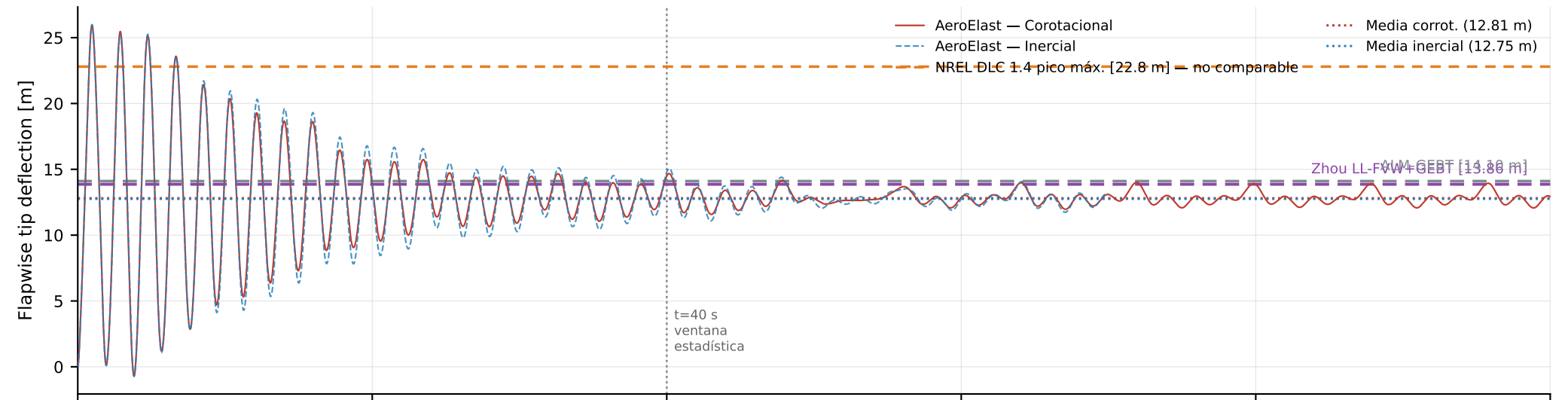
(a) Deflexión flapwise — tip de pala, yaw=0°, condición rated
