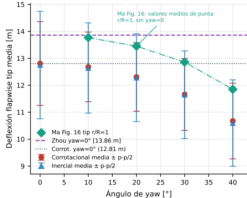
Deflexión flapwise tip — medias
