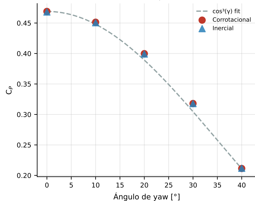
Coeficiente de potencia
