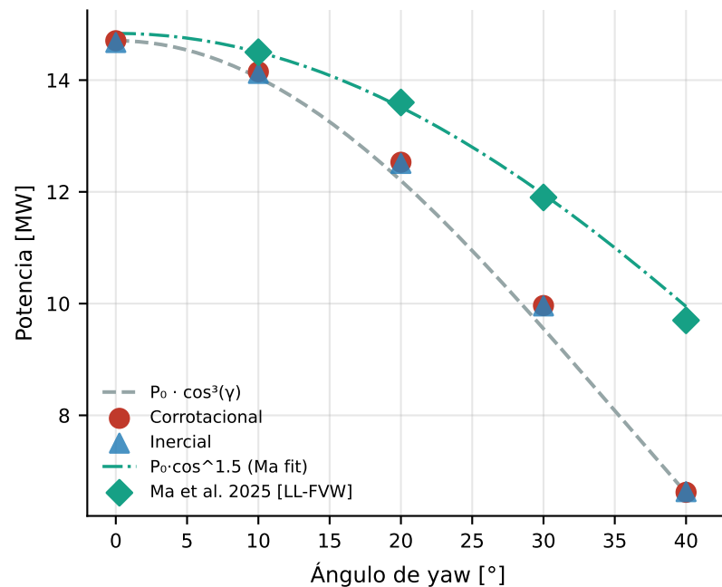
Potencia aerodinámica
