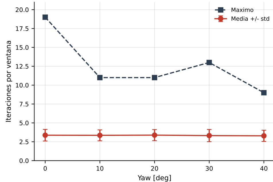
Subiteraciones preCICE
