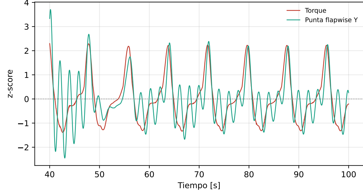
(d) Fluctuación de torque vs fluctuación flapwise
