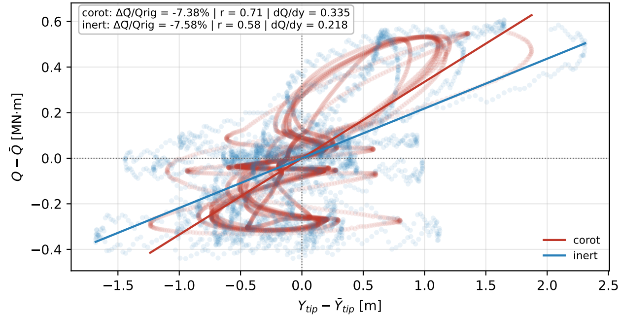
(d) Fluctuación de torque vs fluctuación flapwise
