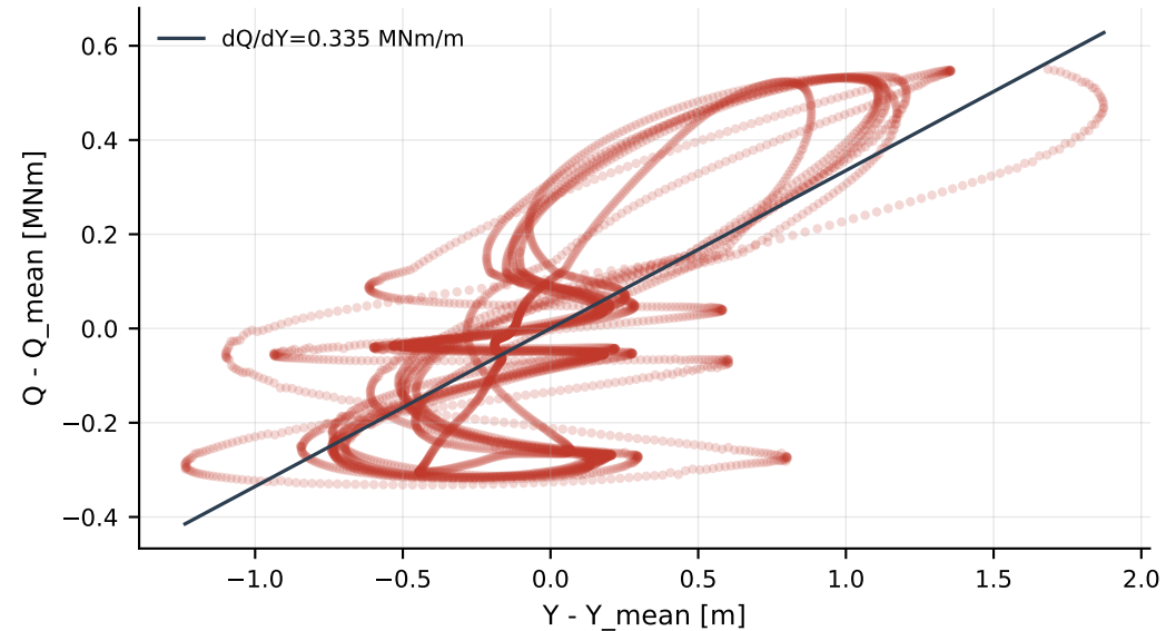
(d) Centered torque vs centered flapwise
