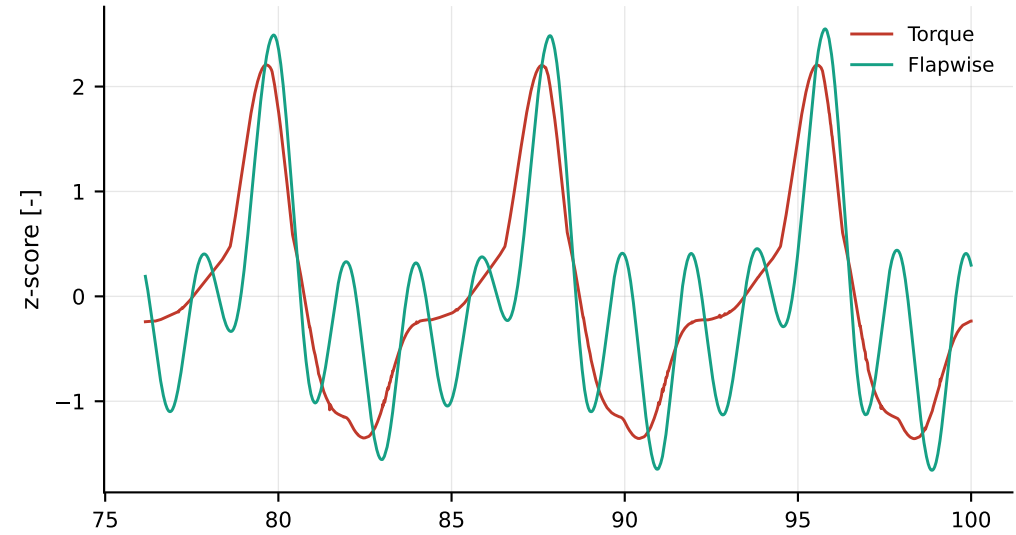
(d) Centered torque vs centered flapwise
