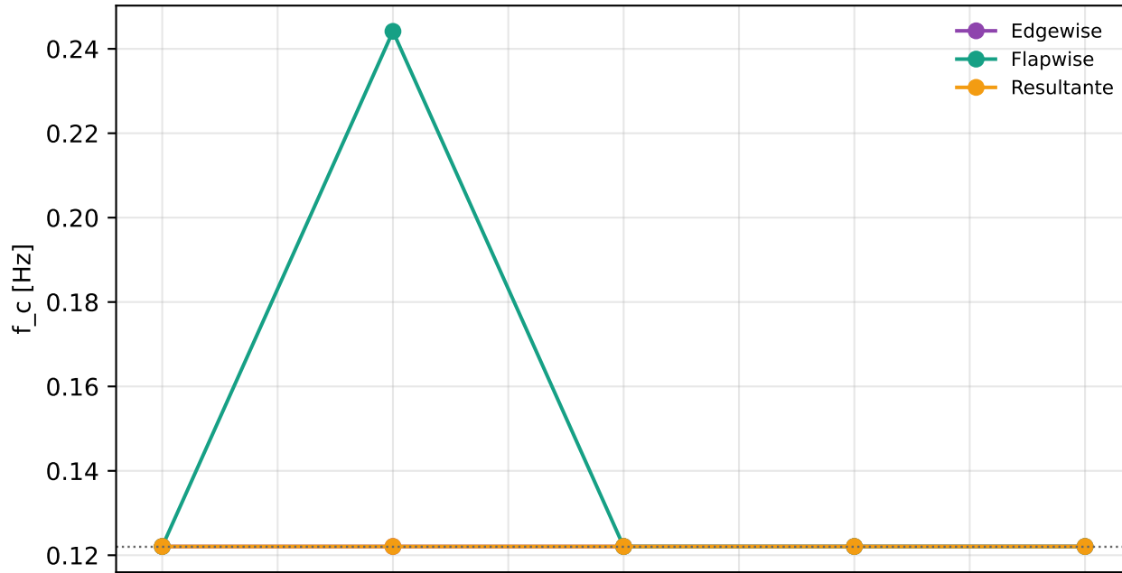
(a) Corrotacional: frecuencia de maximo copoder
