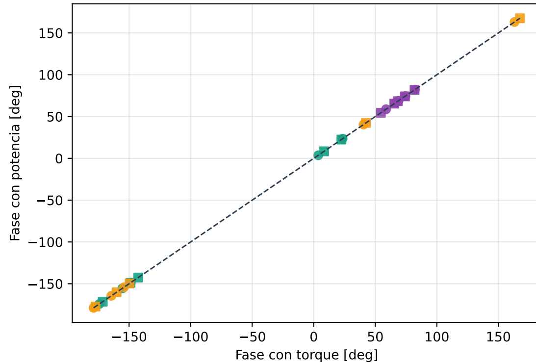
(d) Fase: potencia vs torque
