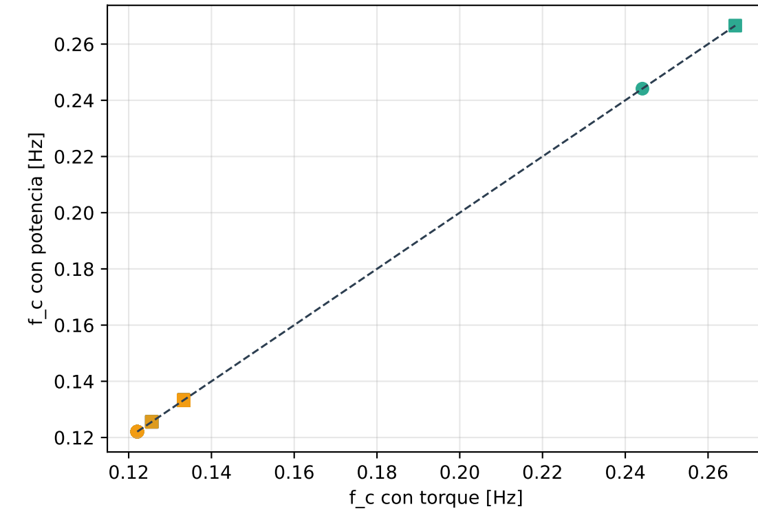
(c) Frecuencia de acoplamiento: potencia vs torque
