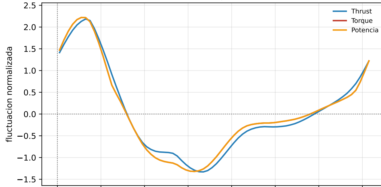
(c) Inercial: cargas aerodinamicas
