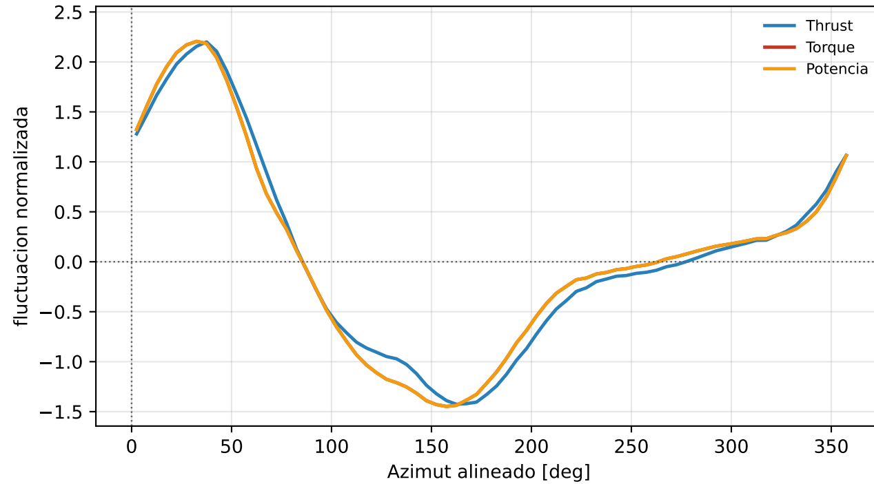
(c) Inercial: cargas aerodinamicas
