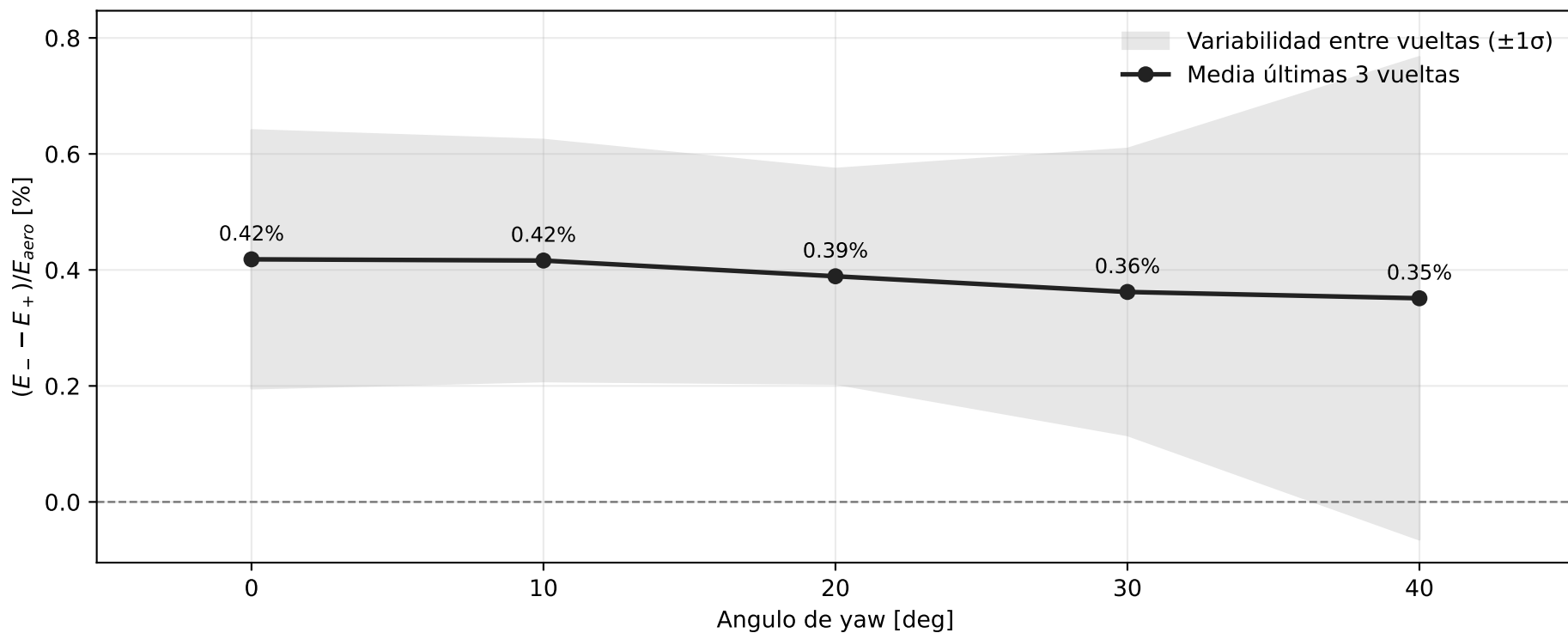
Energía almacenada liberada dentro de la ventana: escala real sobre E_{aero}
