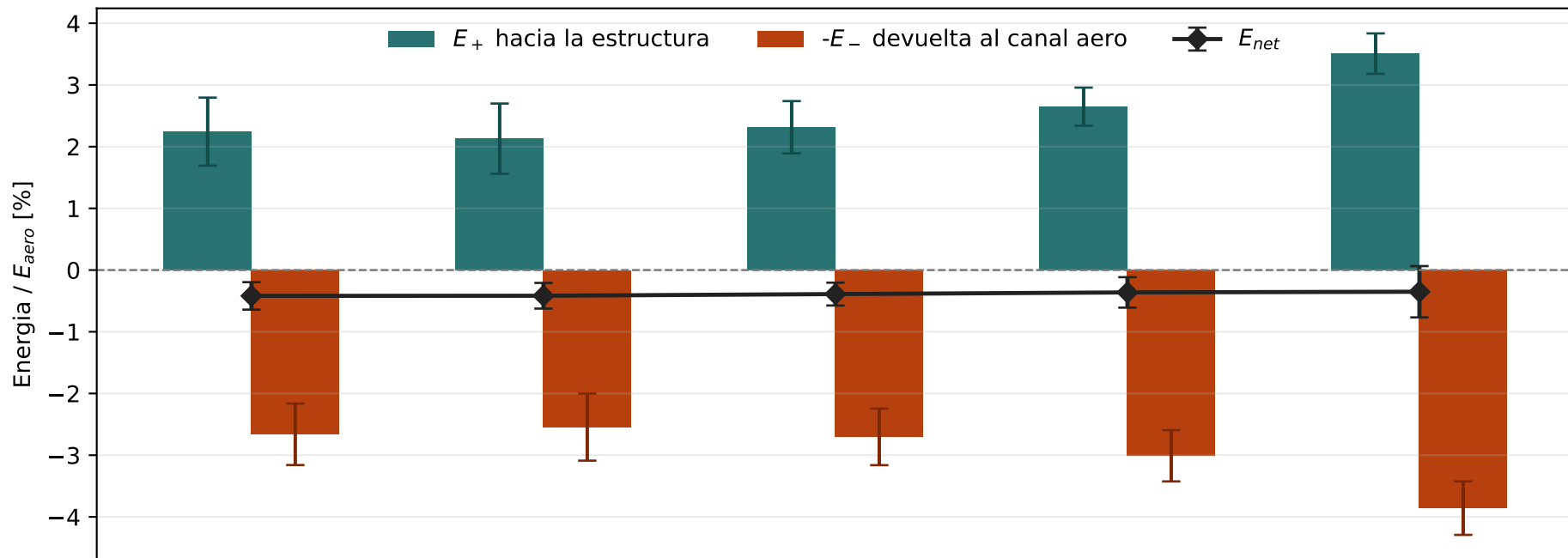
Balance firmado del canal estructural en las ultimas 3 vueltas
