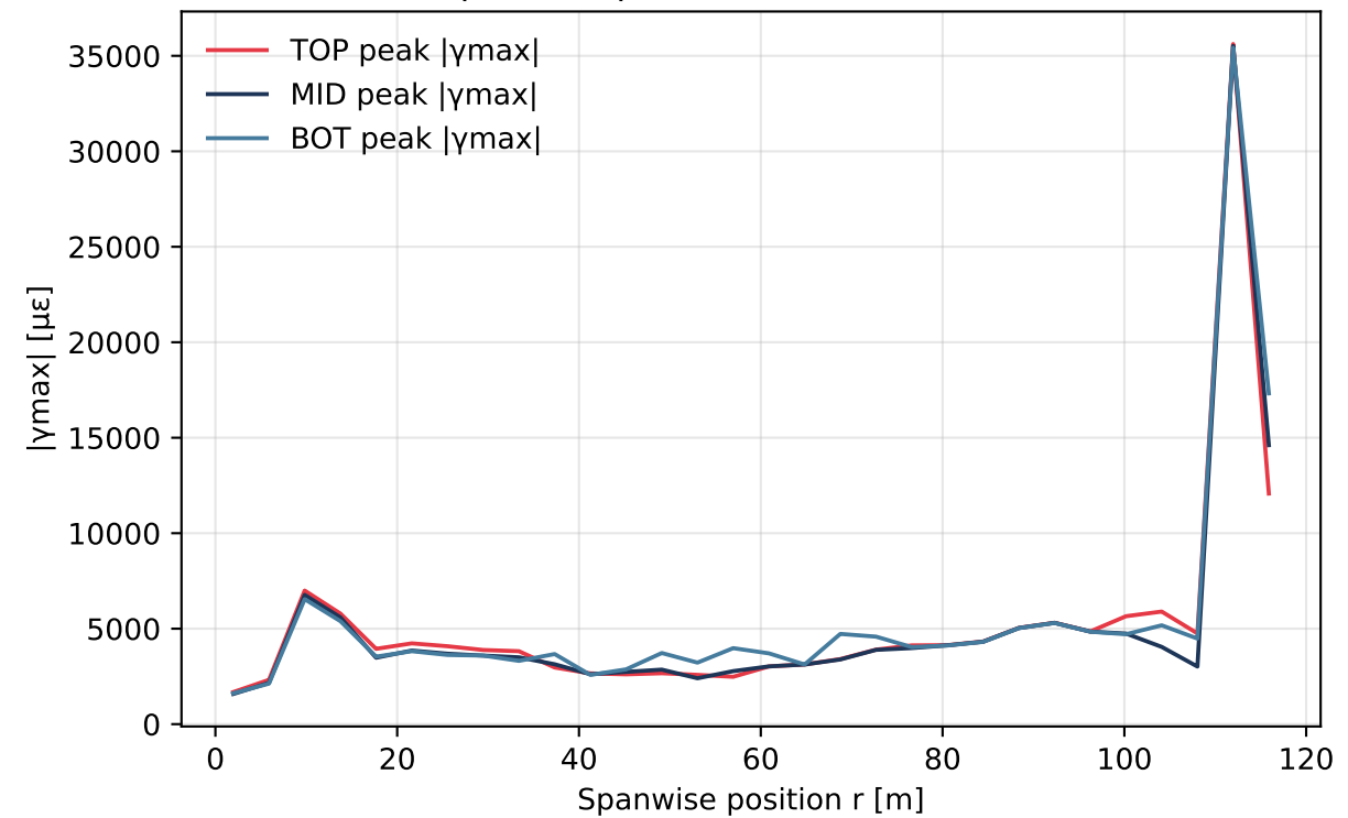
(d) Spanwise peak shear strain (30 bands)
