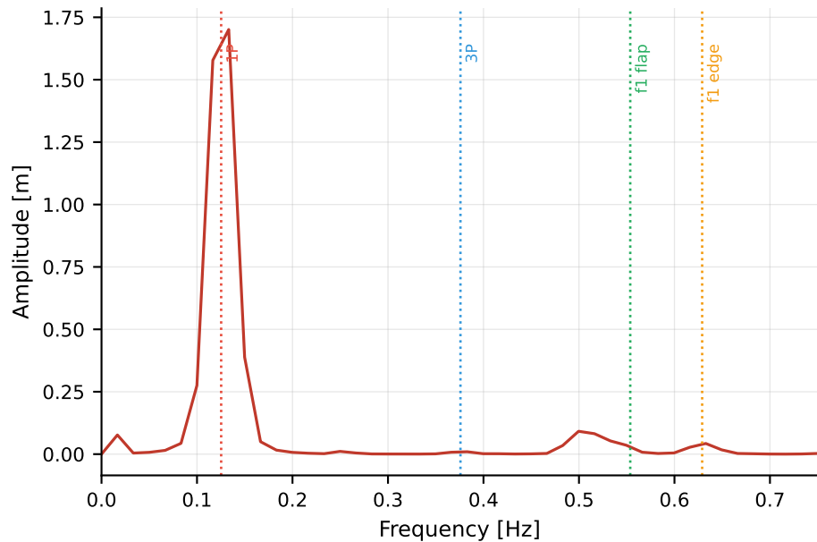
(b) Edgewise tip FFT
