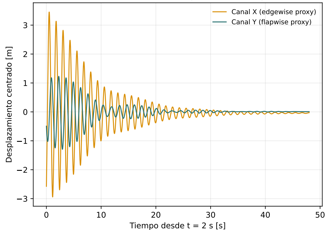
Oscilacion residual despues de la rampa
