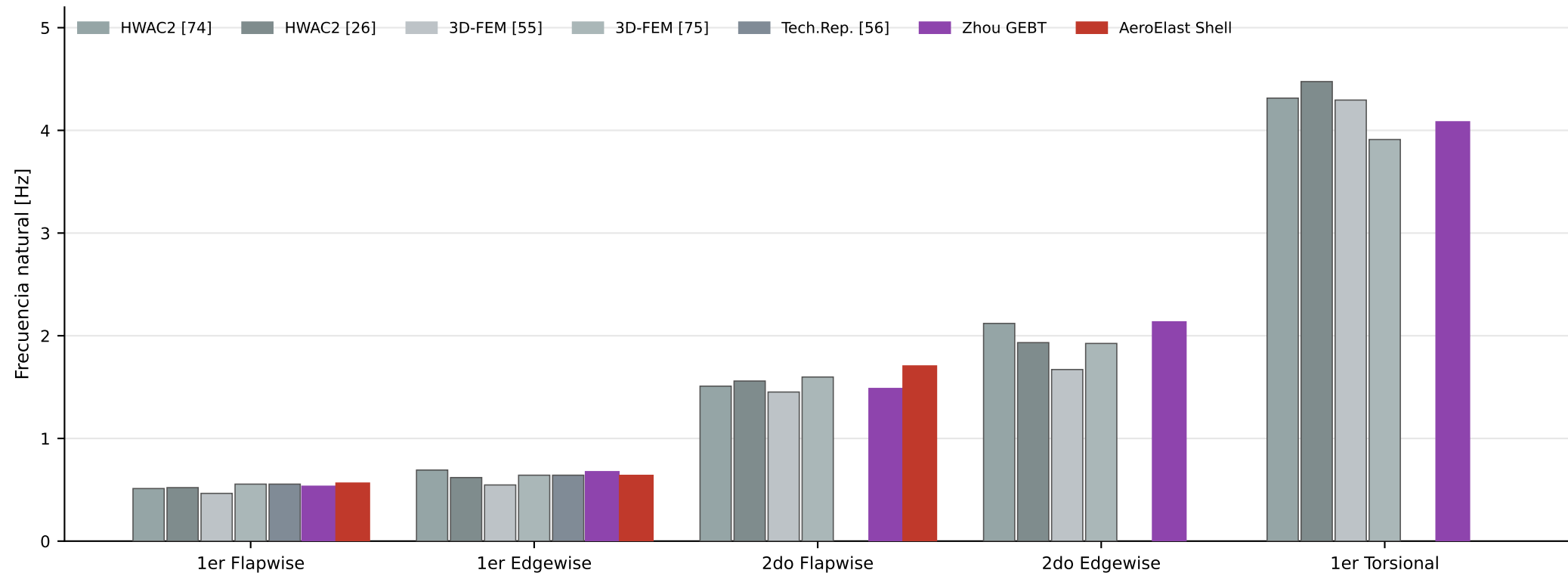
Frecuencias naturales de la pala IEA 15 MW — comparación multi-método (Fuente: Zhou et al. Energy 2025, Tabla 3)
