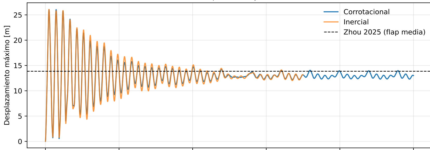
Serie temporal FSI, yaw=0°
