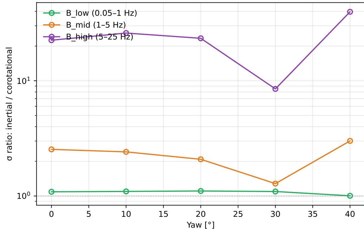
Ratio inercial/corot por banda y por yaw
