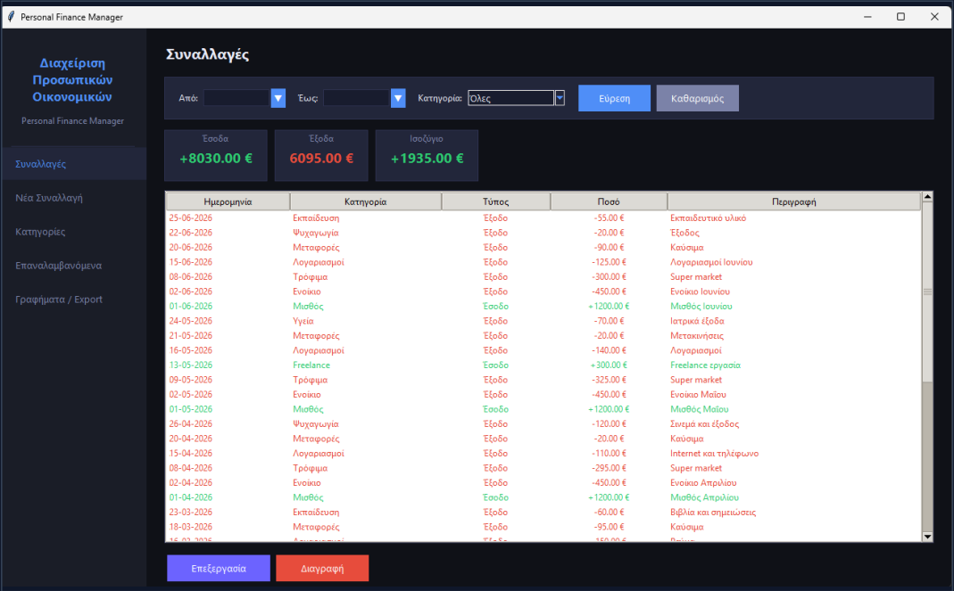
Desktop εφαρμογή σε Python / Tkinter / SQLite
