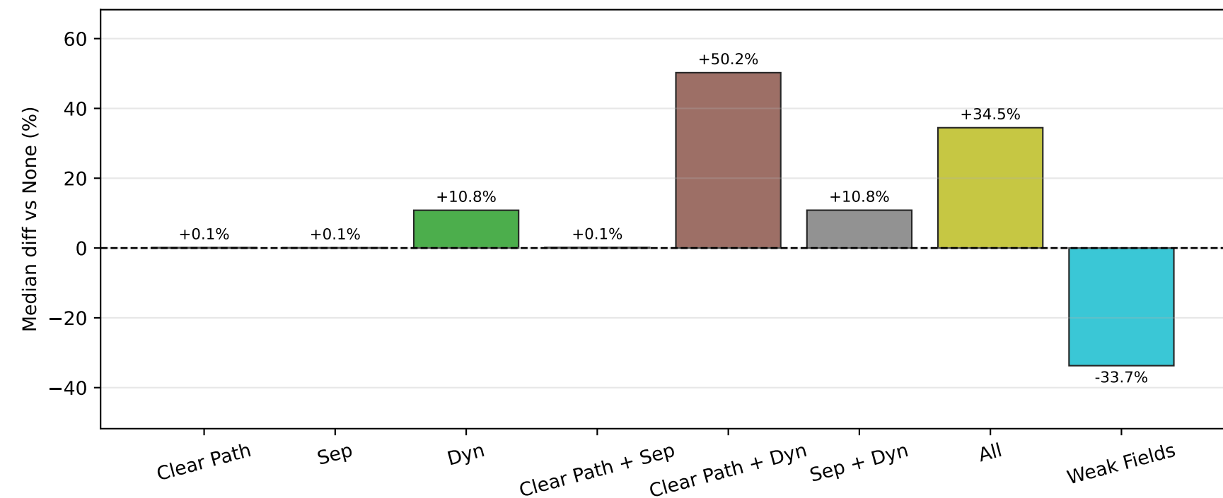
RSS
