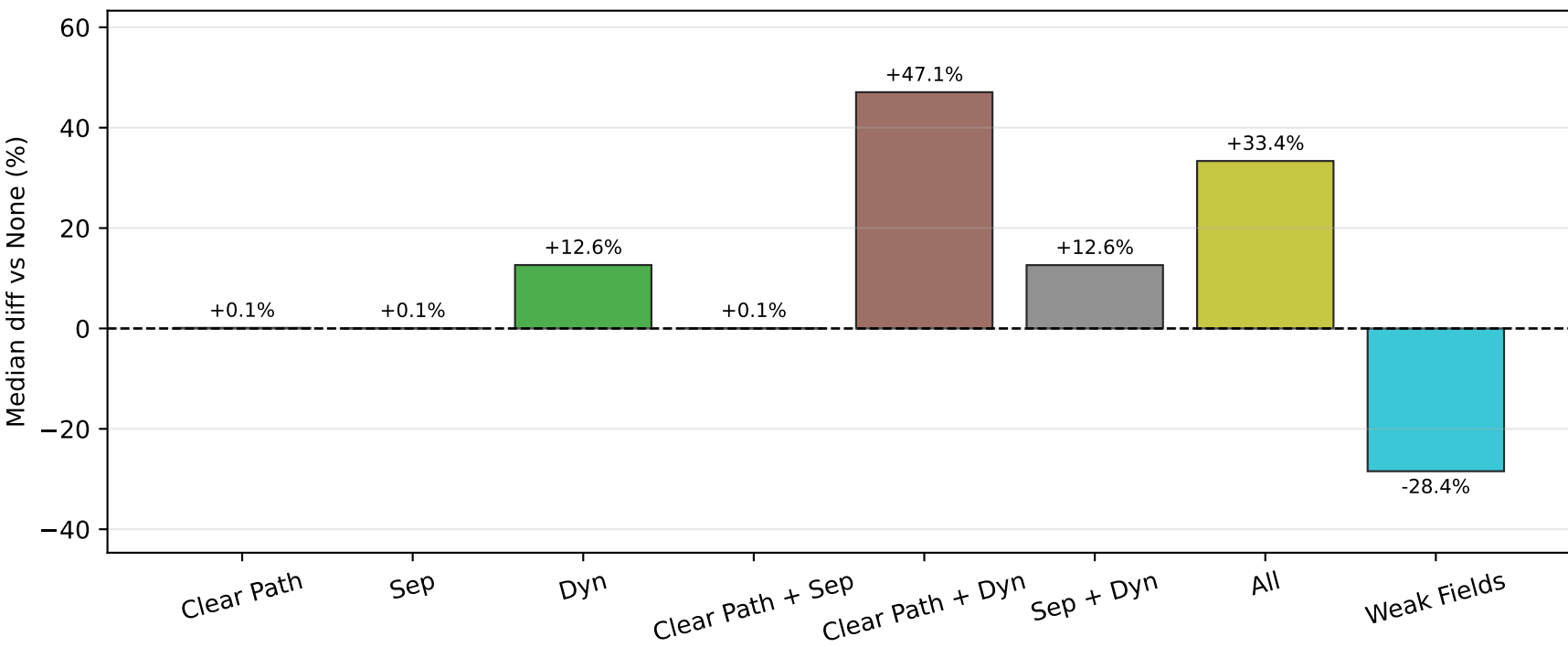
RSS
