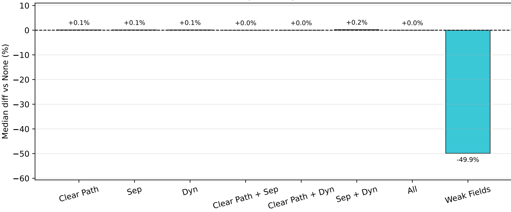
RSS
