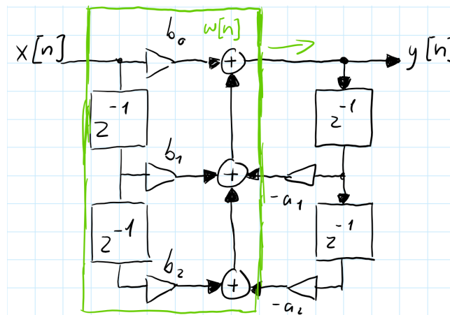
Abbildung 16.1.: Signalflussbild: Direktform 1
