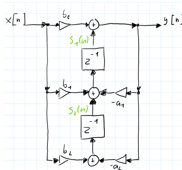
Abbildung 0.3: Signalflussbild: Transponierte Direktform 2
