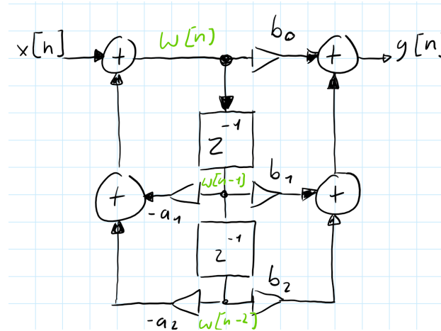
Abbildung 0.2: Signalflussbild: Direktform 2
