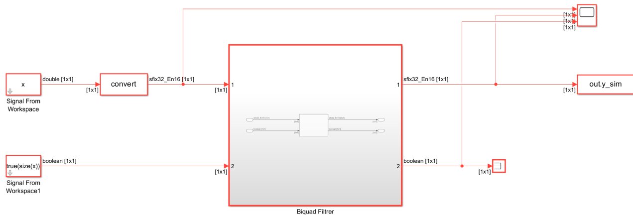
Abbildung 23.3.: Simulink Filter
