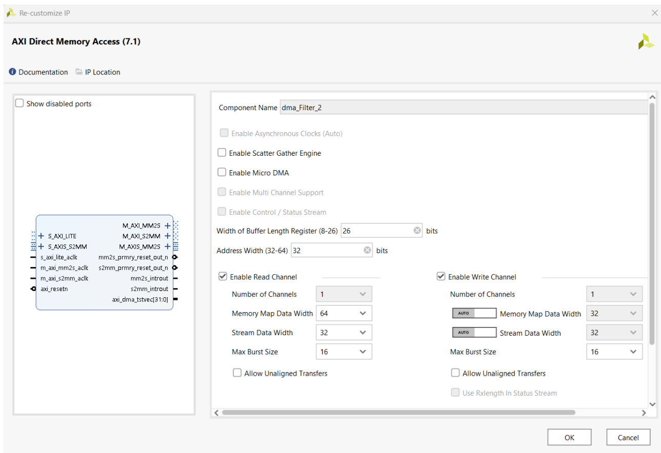
Abbildung 18.12.: AXI-DMA Config
