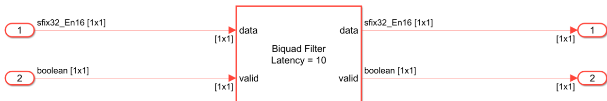
Abbildung 18.1.: Simulink Filter: Subsystem
