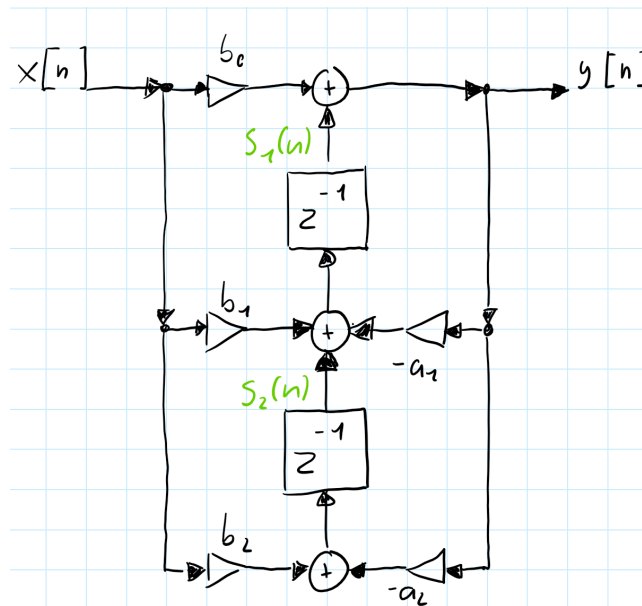
Abbildung 15.3.: Signalflussbild: Transponierte Direktform 2
