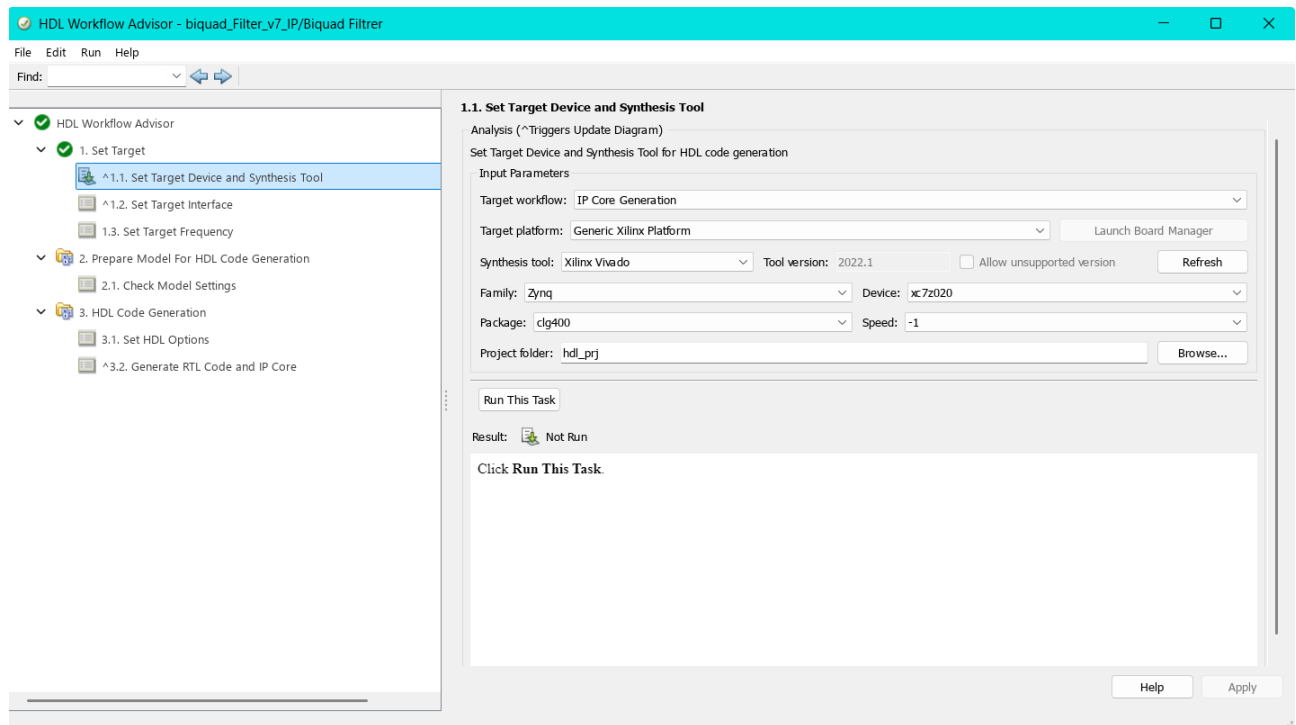
Abbildung 18.4.: HDL Workflow: Target Device
