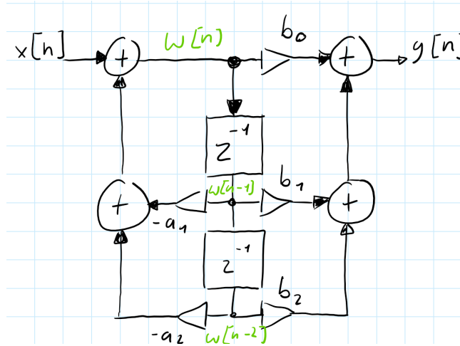
Abbildung 15.2.: Signalflussbild: Direktform 2
