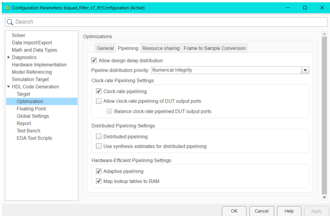
Abbildung 18.7.: HDL Workflow: HDL Options/ Optimization/ Pipelining
