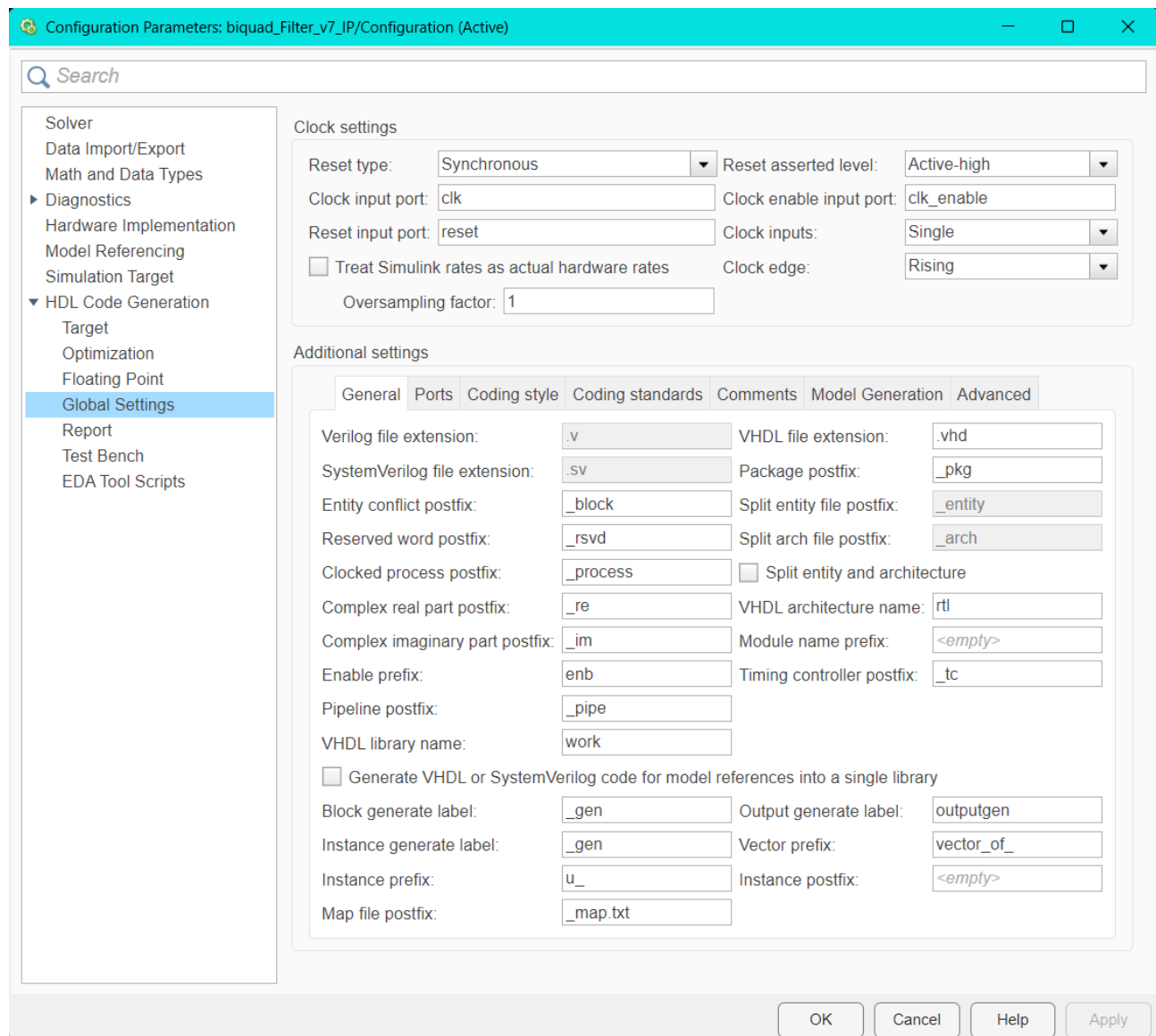
Abbildung 18.8.: HDL Workflow: HDL Options/ Global Settings
