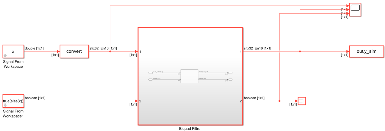
Abbildung 18.3.: Simulink Filter
