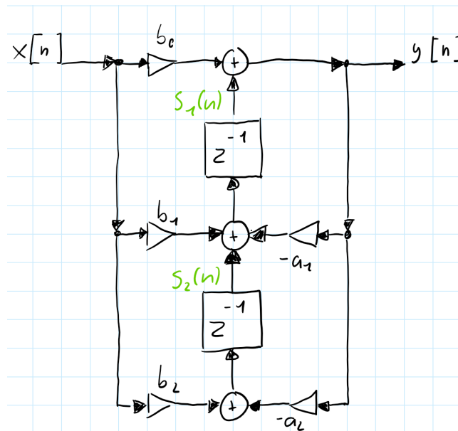
Abbildung 18.3.: Signalflussbild: Transponierte Direktform 2
