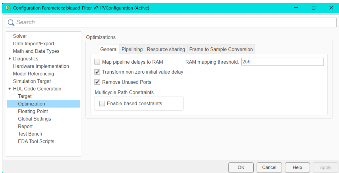
Abbildung 22.6.: HDL Workflow: HDL Options/ Optimization/ General
