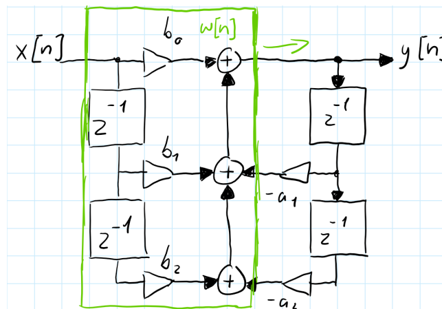
Abbildung 18.1.: Signalflussbild: Direktform 1
