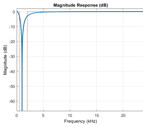
(b) Digitaler Butterworth-Bandstopfilter 2. Ordnung
