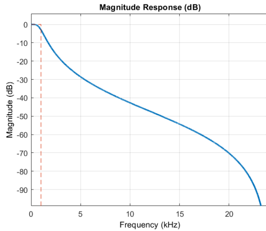
(b) Digitaler Butterworth-Tiefpassfilter 2. Ordnung
