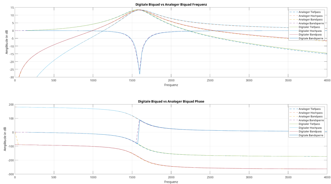
Abbildung 10.2.: Vergleich zwischen analogen und digitalen Frequenz- und Phasengang
