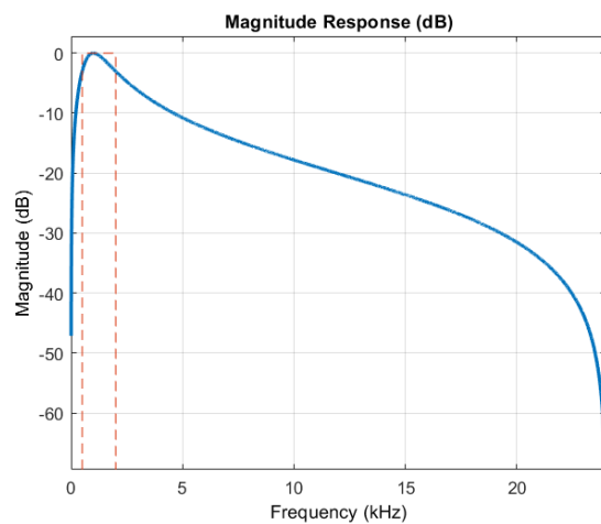
(a) Digitaler Butterworth-Bandpassfilter 2. Ordnung
