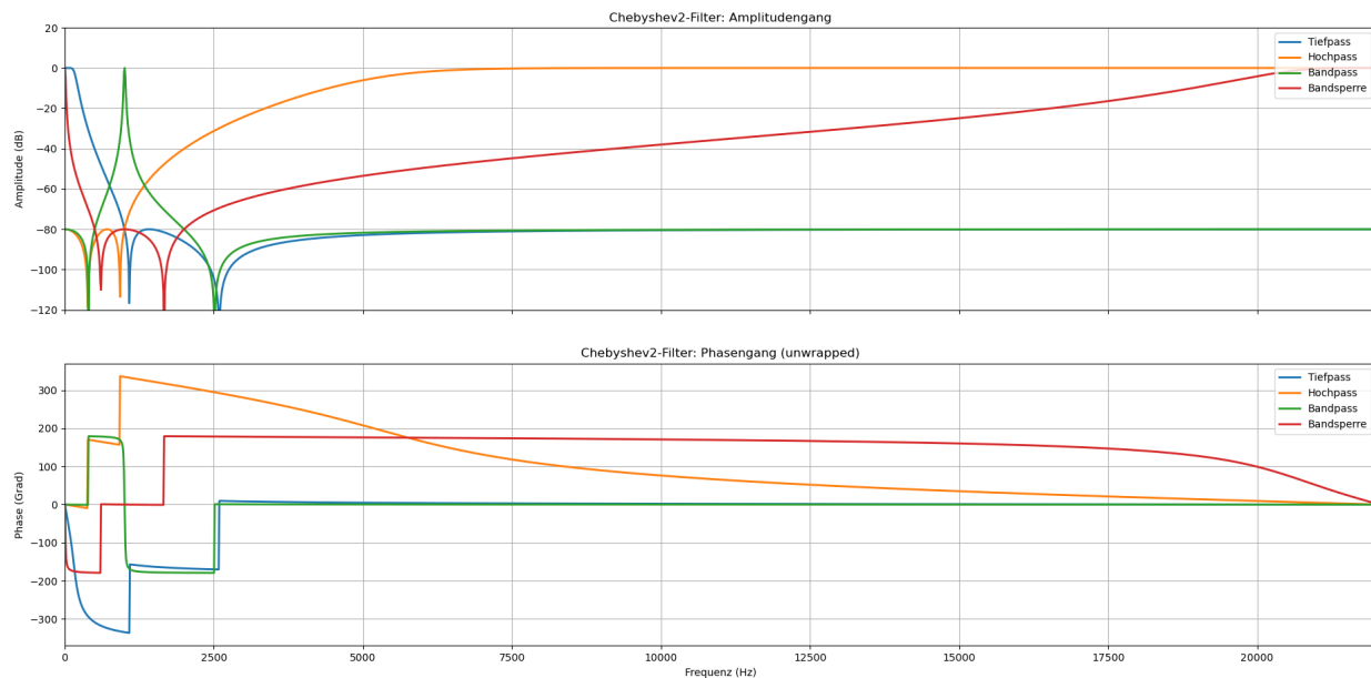
Abbildung 11.3.: Chebyshev2-Filter
