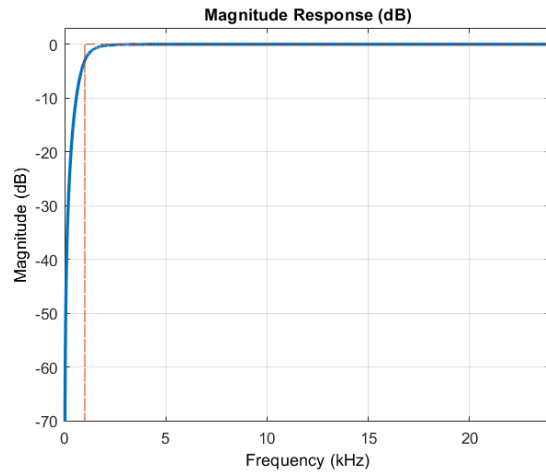
(a) Digitaler Butterworth-Hochpassfilter 2. Ordnung
