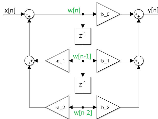
Abbildung 20.2.: Signalflussbild: Direktform 2
