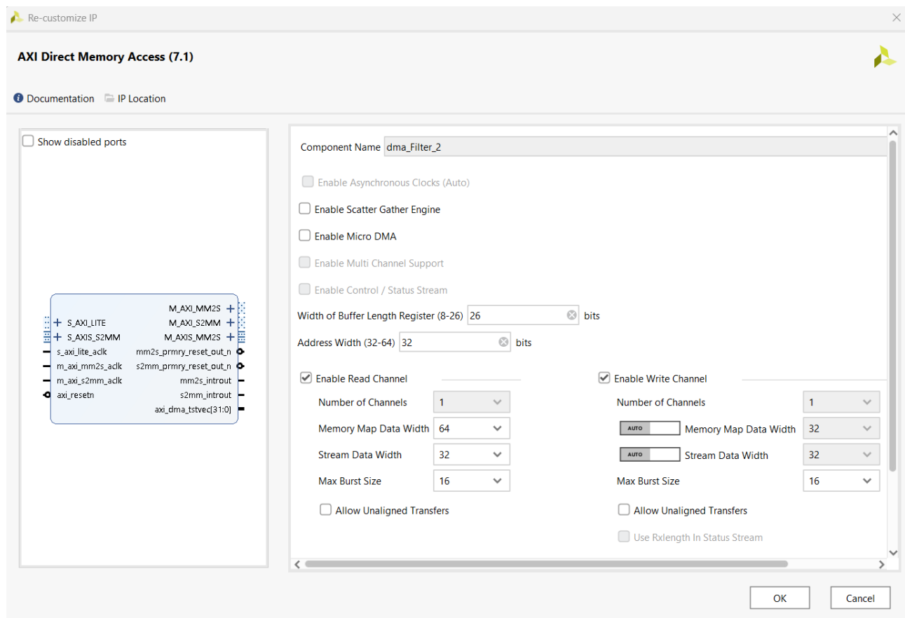
Abbildung 24.12.: AXI-DMA Config
