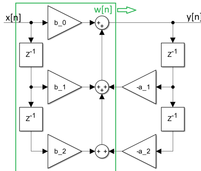
Abbildung 20.1.: Signalflussbild: Direktform 1
