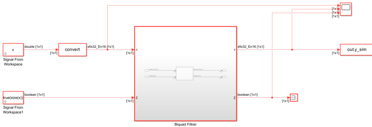
Abbildung 0.3: Simulink Filter
